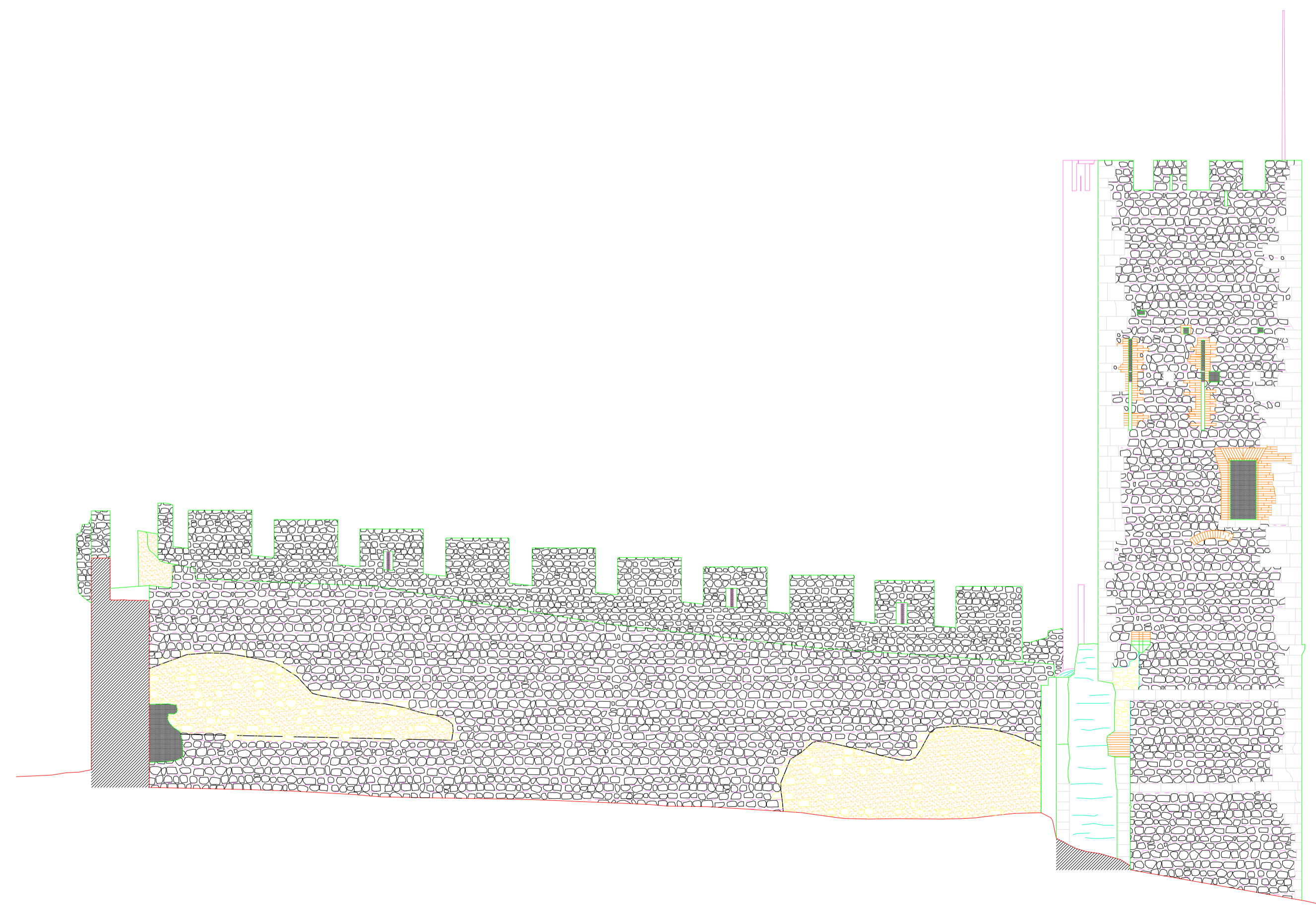
ALÇADO ESTE - INTERIOR
