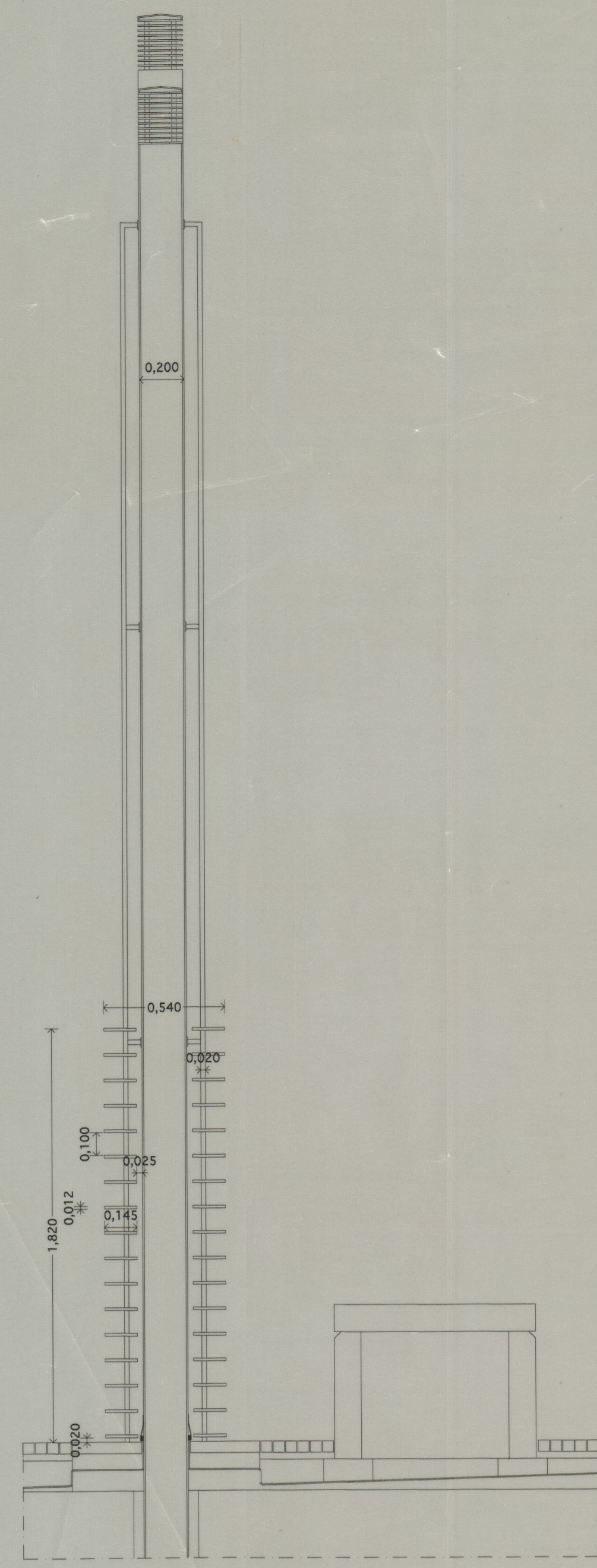
CORTE TRANSVERSAL
