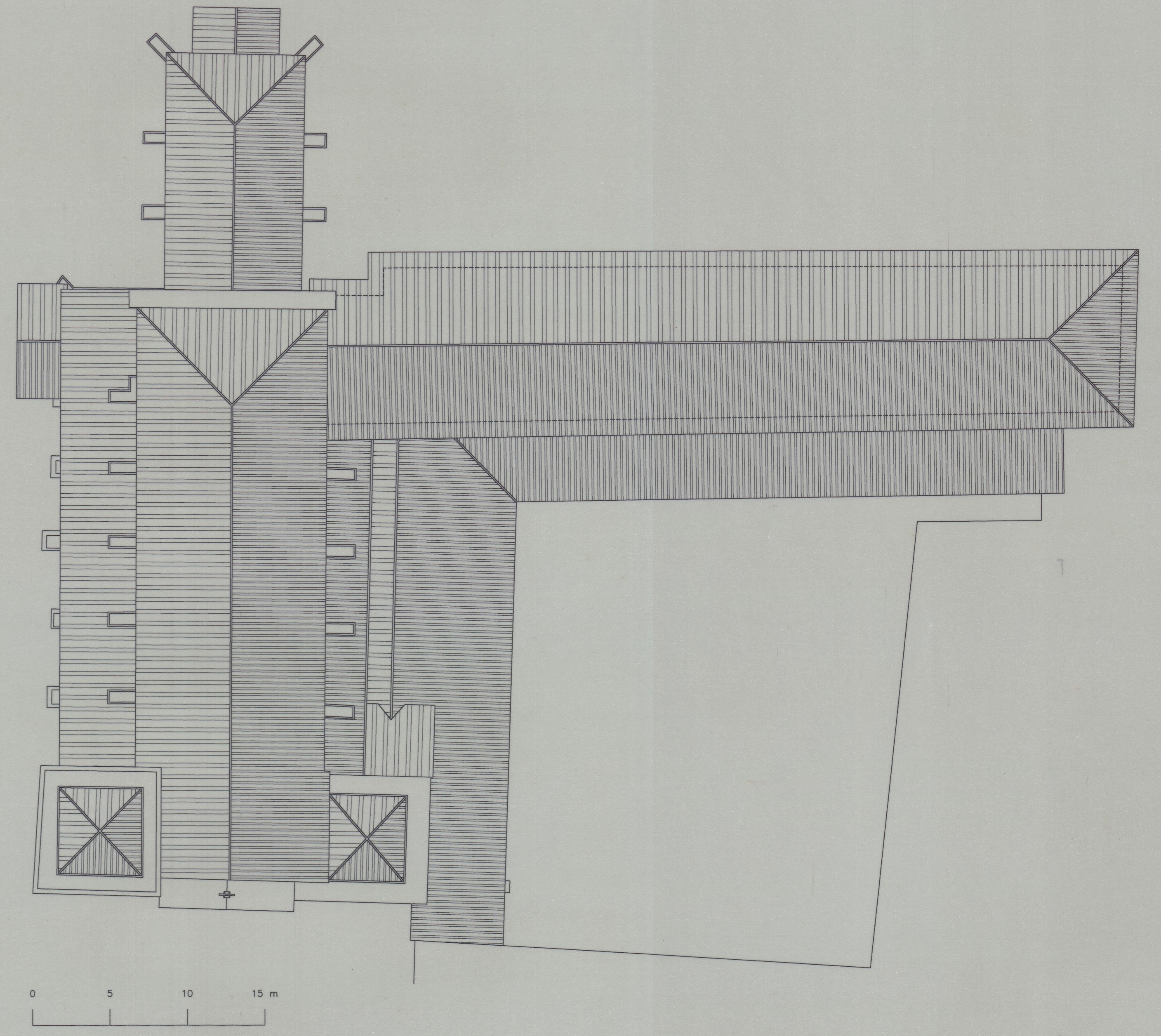
PLANTA DE COBERTURAS
