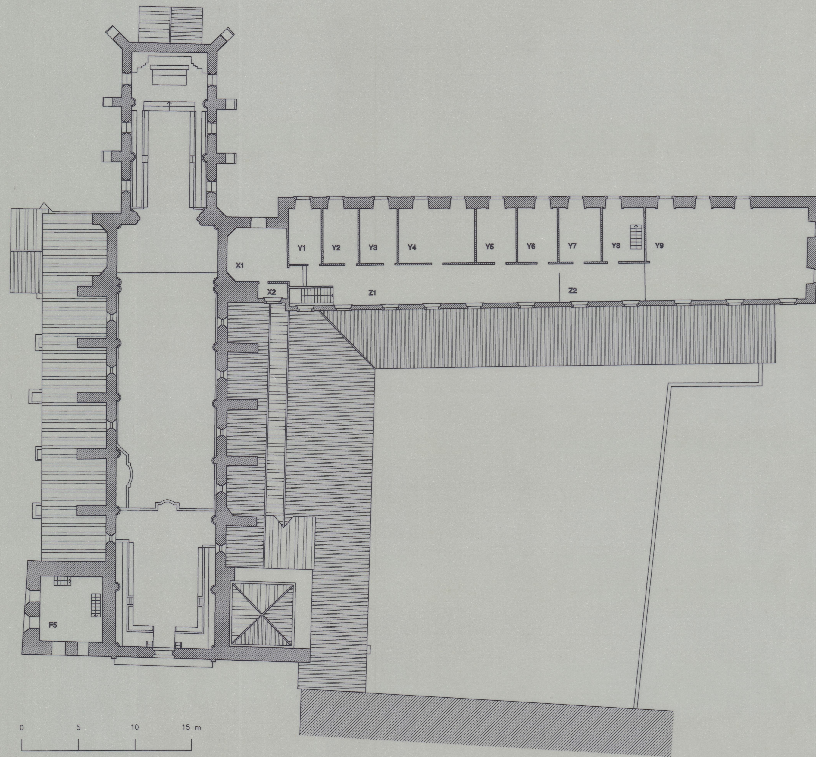
PLANTA DO PISO 2
