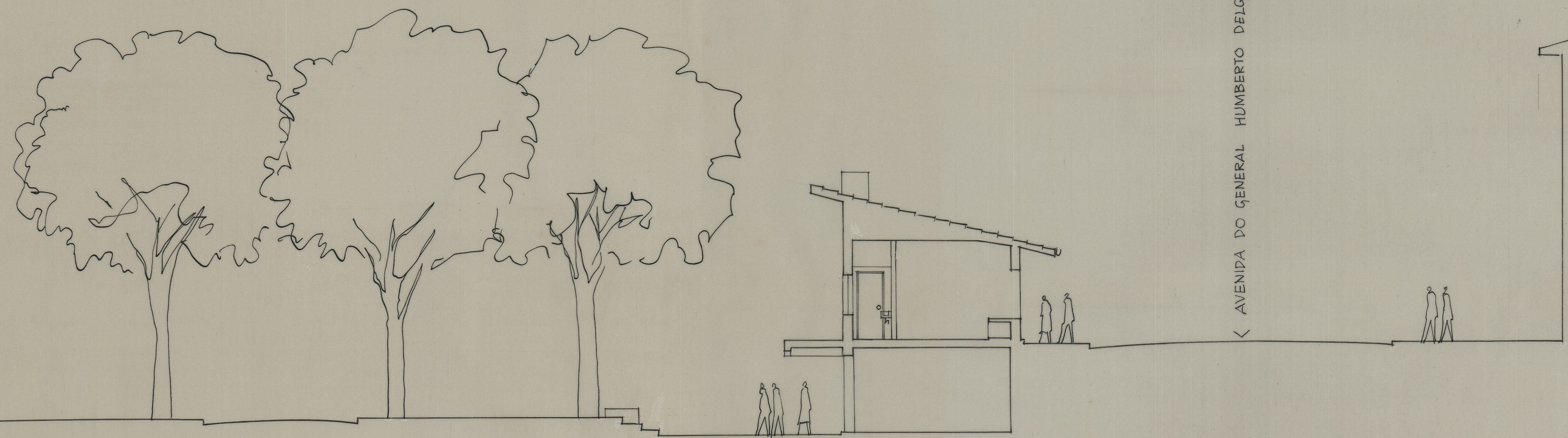
CORTE TRANSVERSAL ESCALA 1/100
