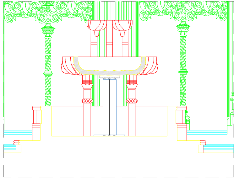
corte pela taça elemento da proposta em alçado
