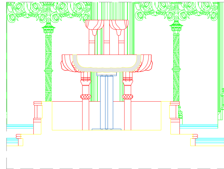
corte pela taça
