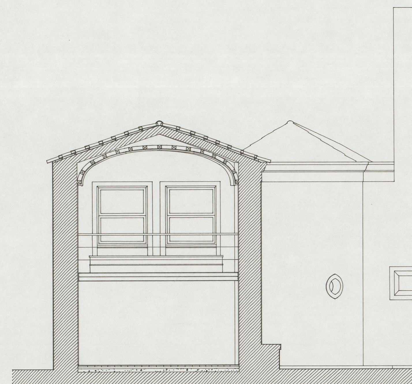
CORTE C6
