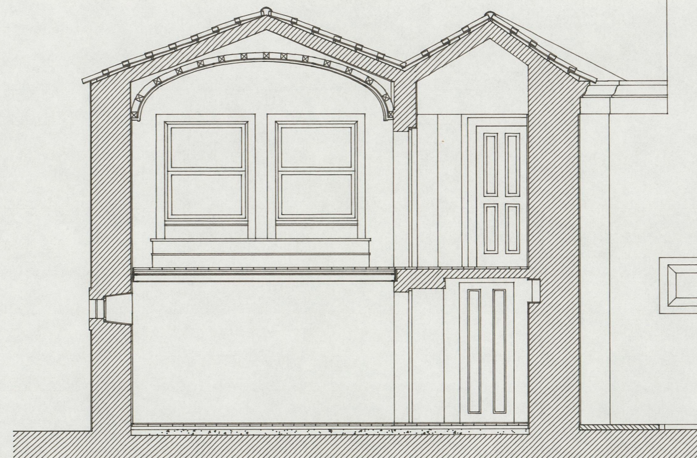
CORTE C7
