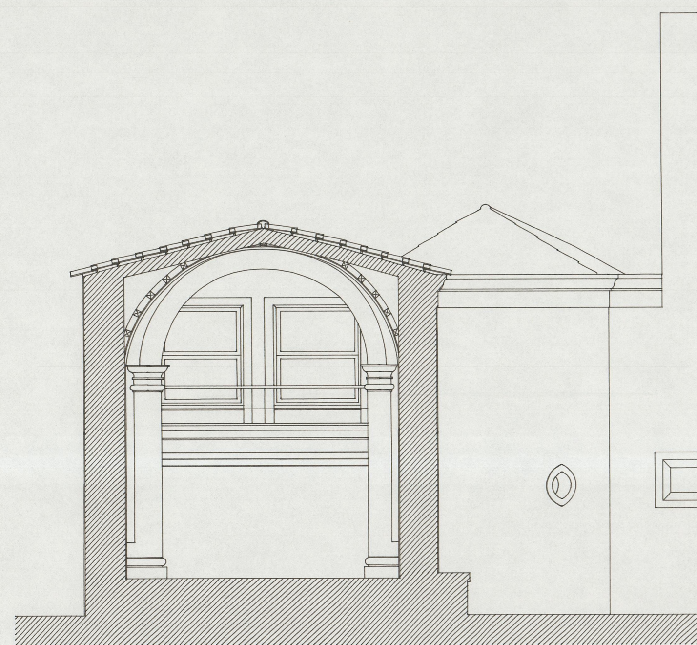
CORTE C3
