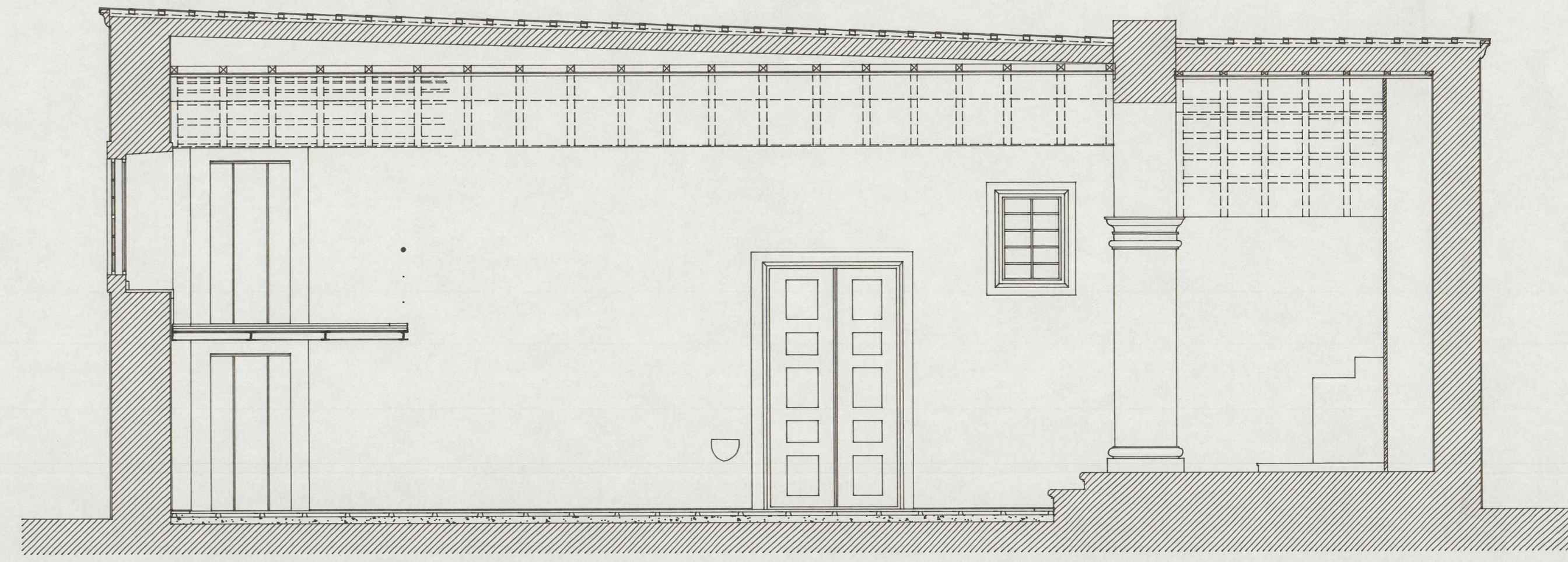
CORTE C2
