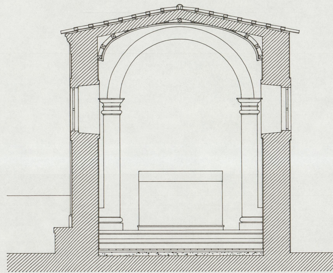
CORTE C4
