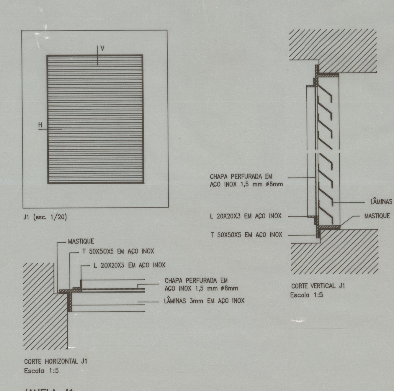
JANELA J1 Escala 1:5
