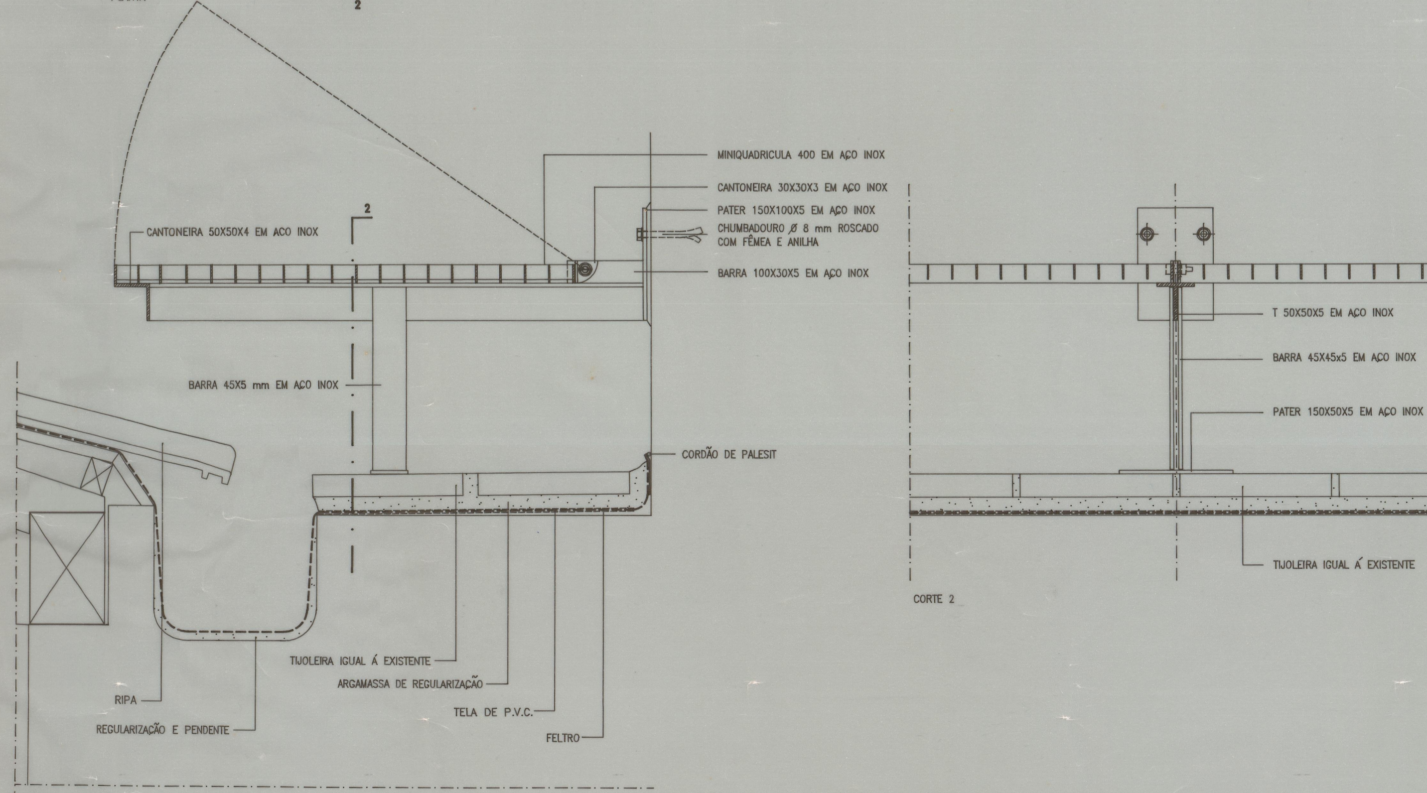
PORM. DA PASSADEIRA EM GRELHA "GRATING" Escala 1:5
