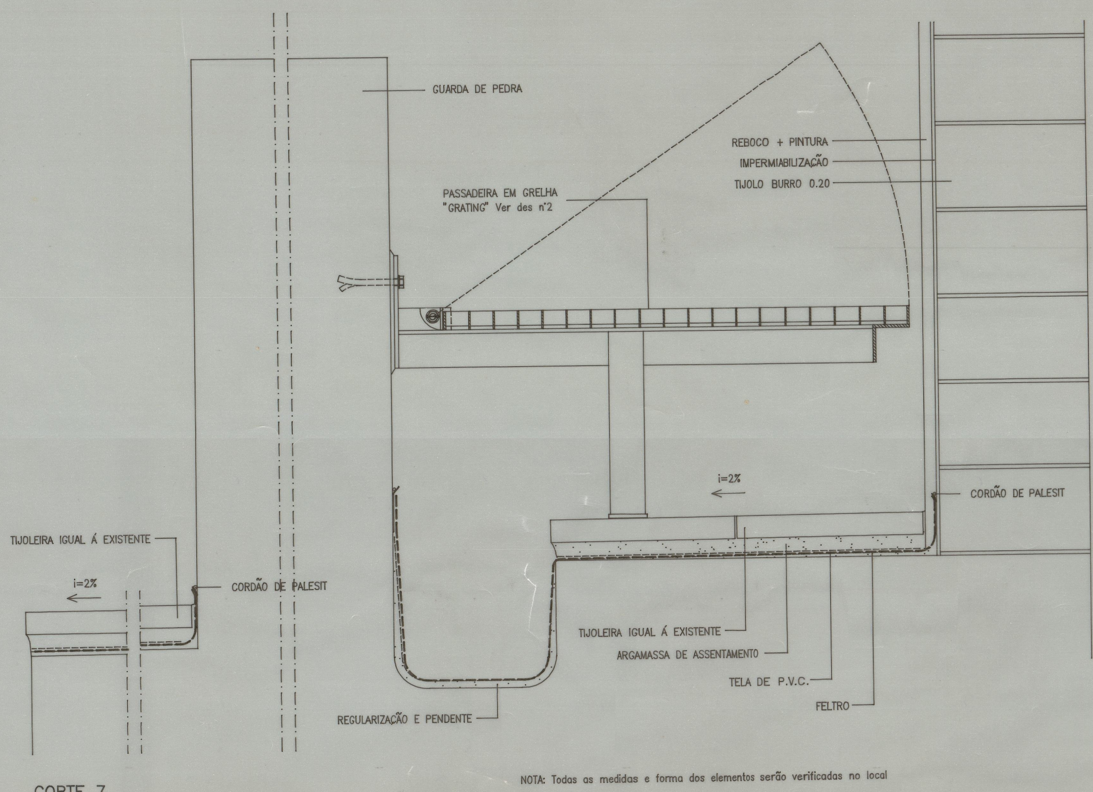
CORTE 7 Escala 1:5
