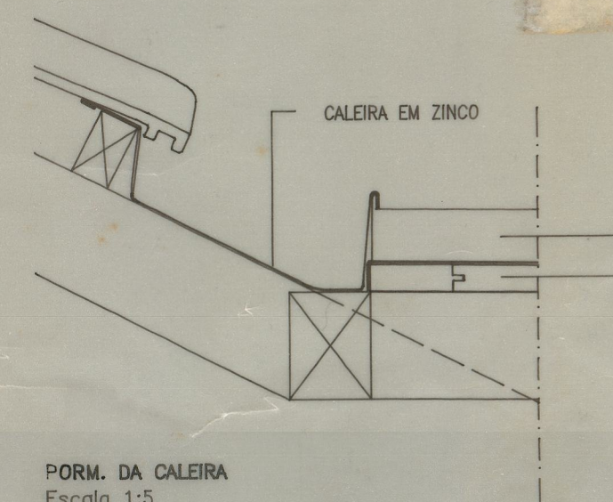
FORM. DA CALERA Escala 1:5
