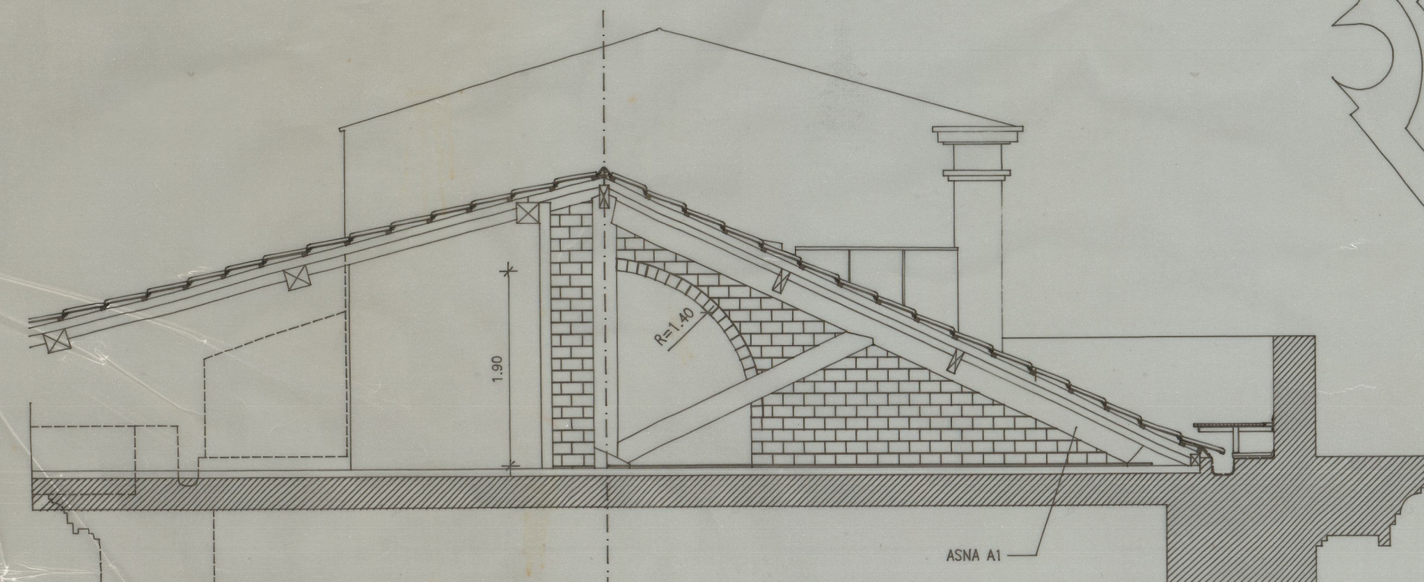
CORTE 1-1 Escala 1:50
