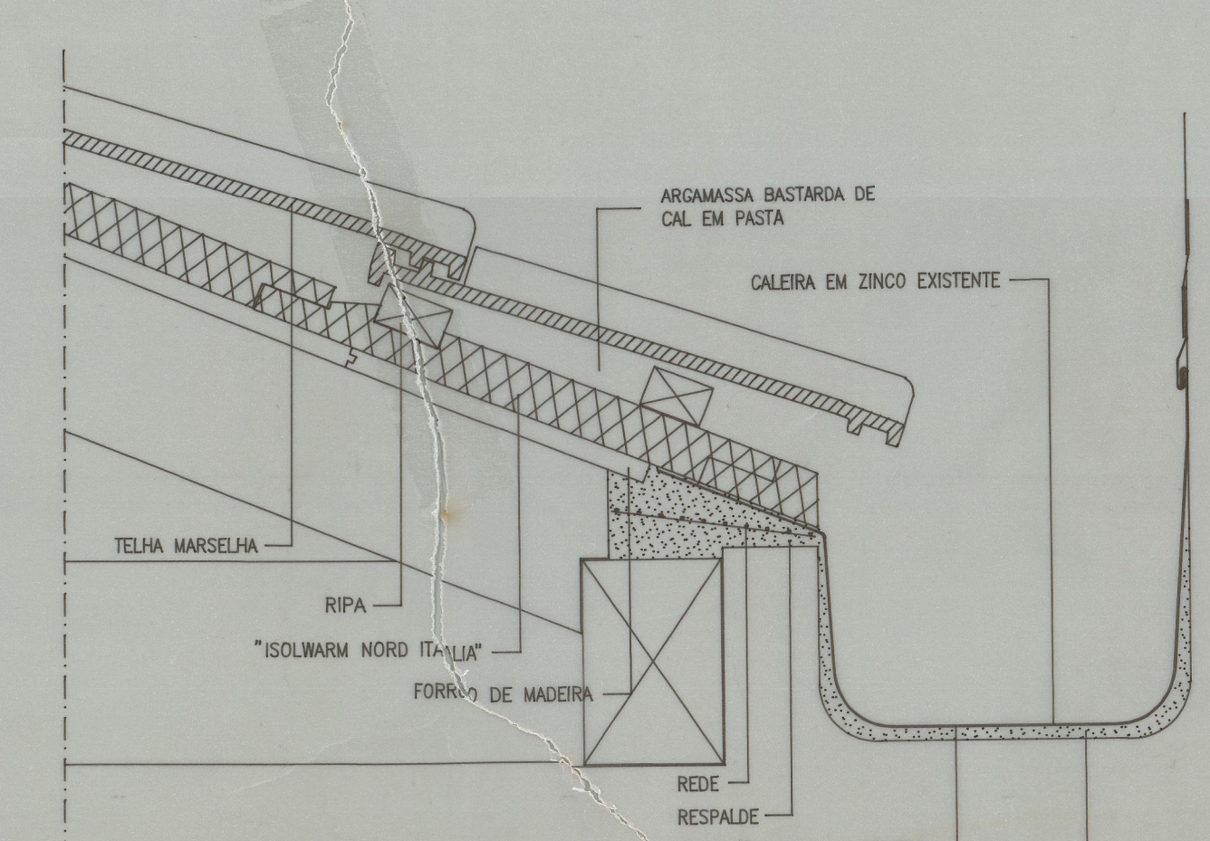
CORTE 6 Escala 1:5
