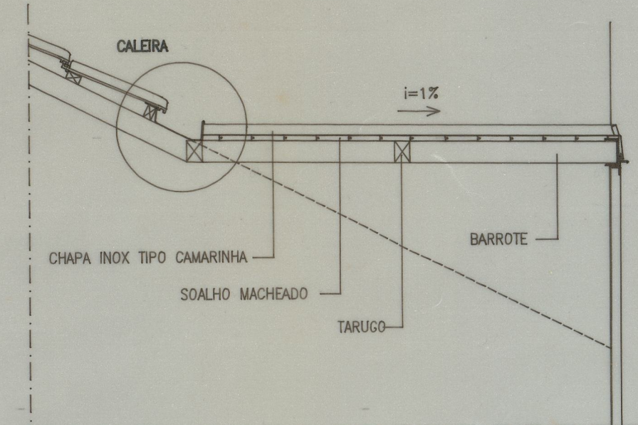
CORTE 3-3 Escala 1:20
