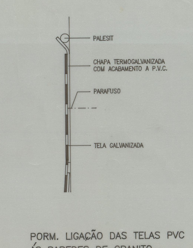
CORTE 7 Escala 1:5
