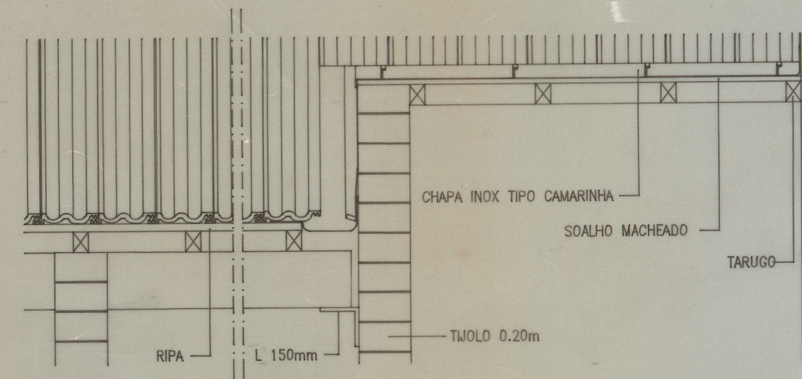
CORTE 2-2 Escala 1:20
