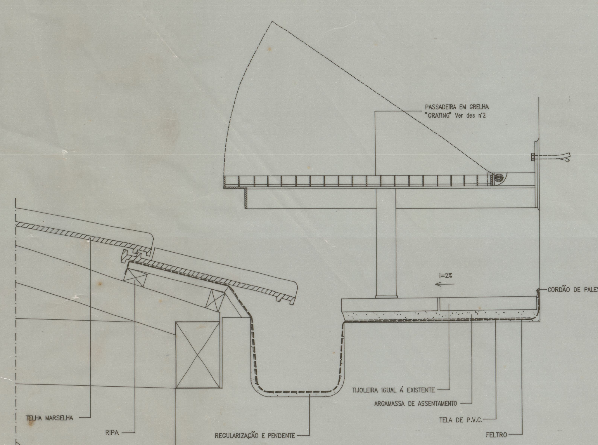
CORTE 4 Escala 1:5
