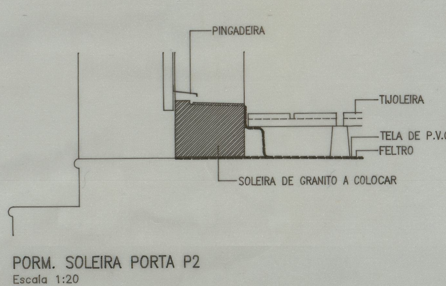
FORM. SOLEIRA PORTA P2 Escala 1:20
