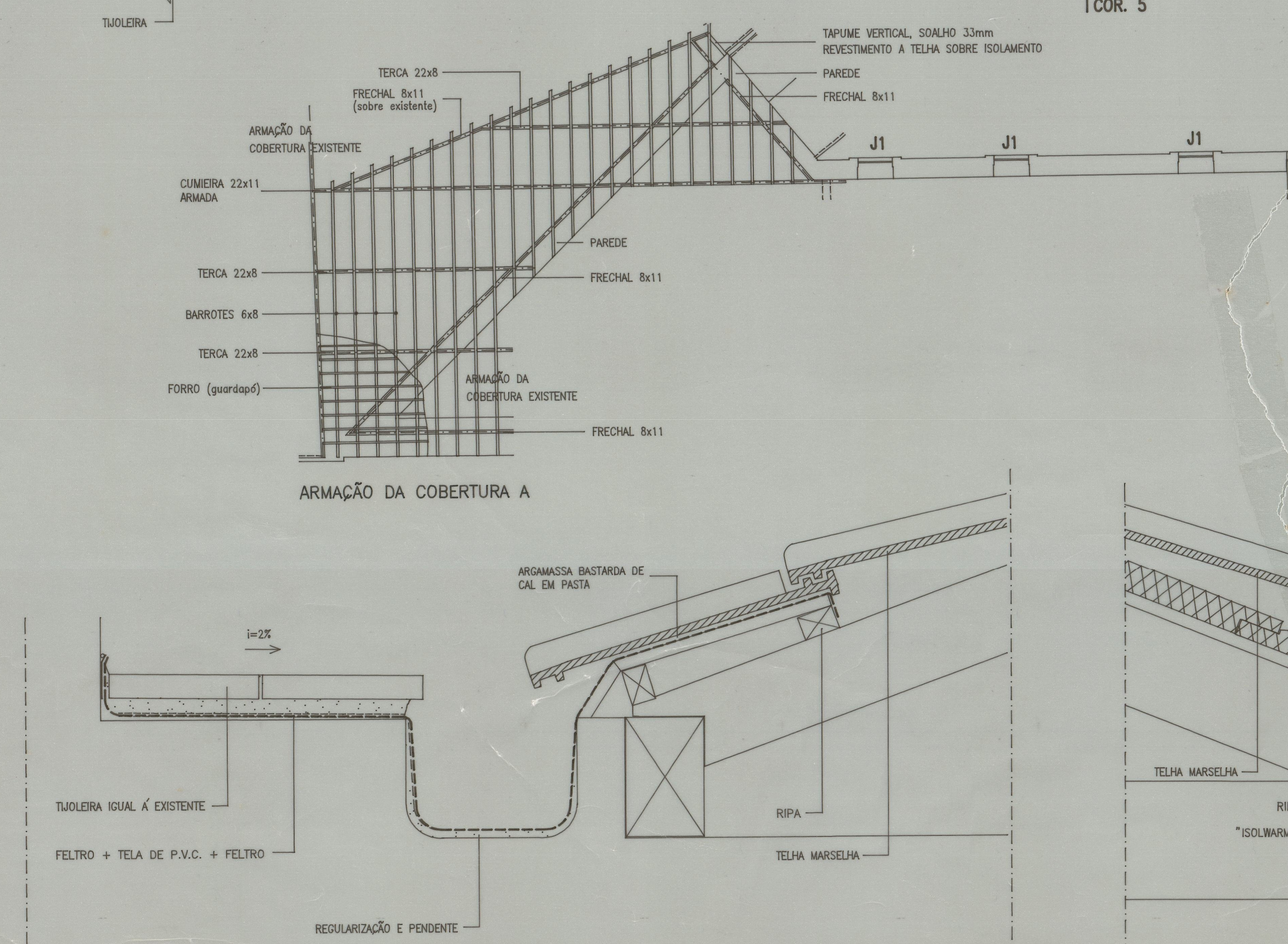
CORTE 5 Escala 1:5
