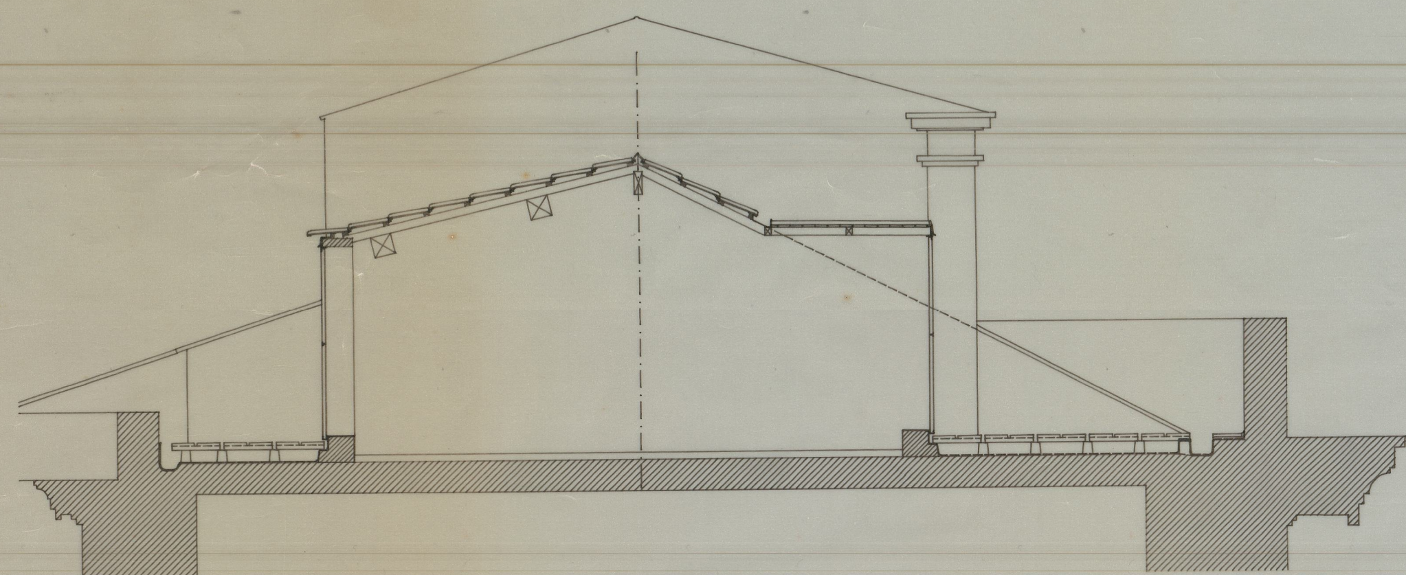
CORTE 2-2 Escala 1:50
