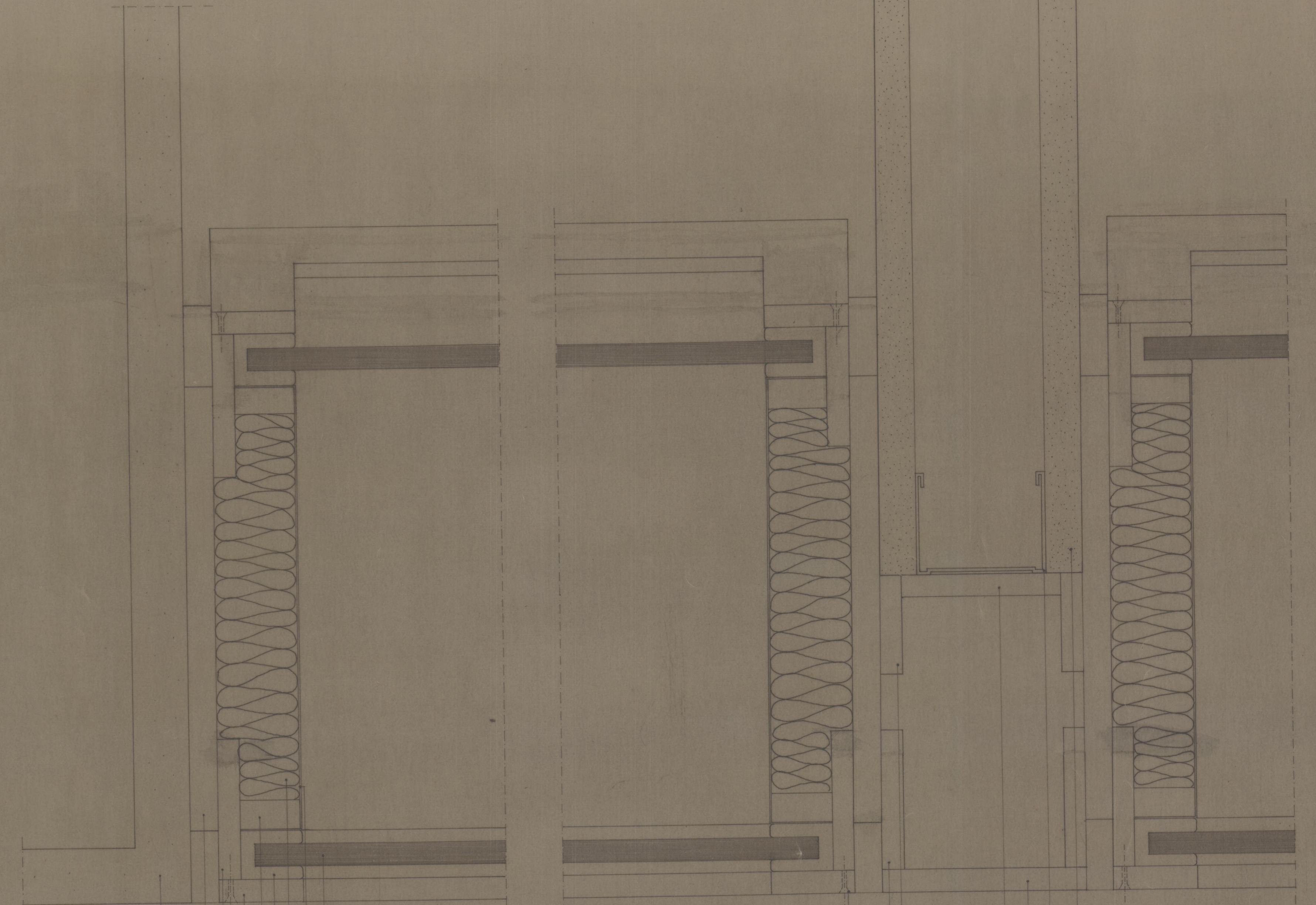
CORTE HORIZONTAL
