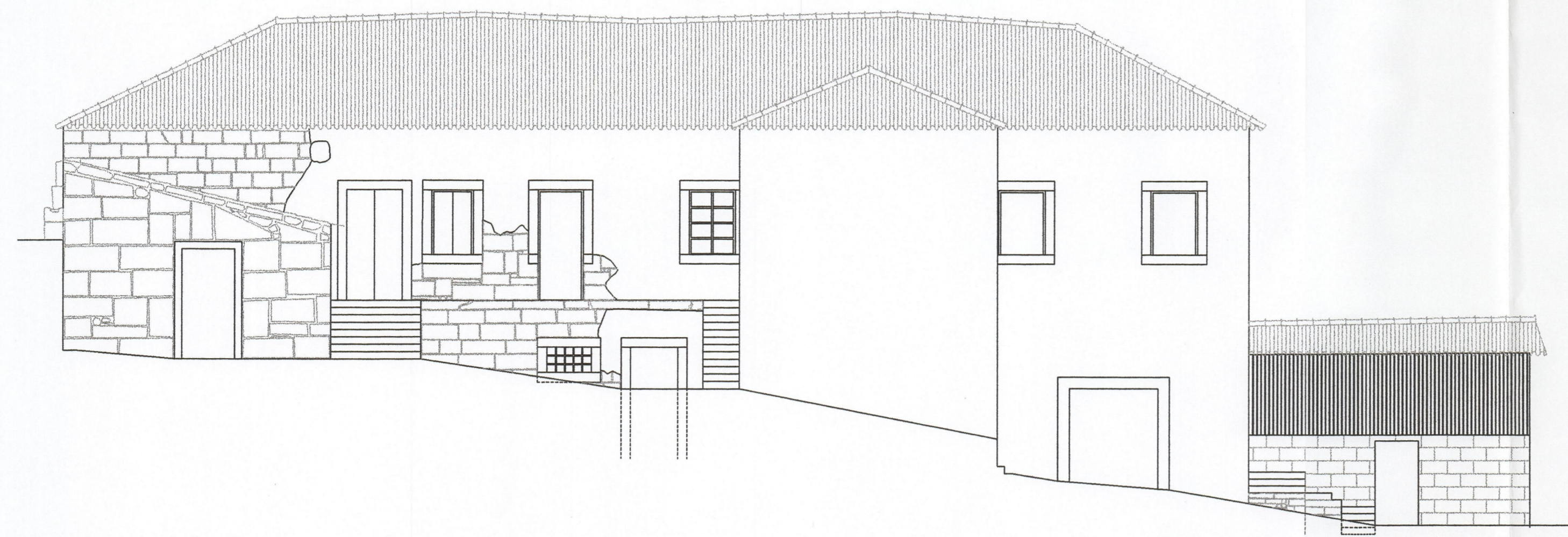
ALÇADO PRINCIPAL
