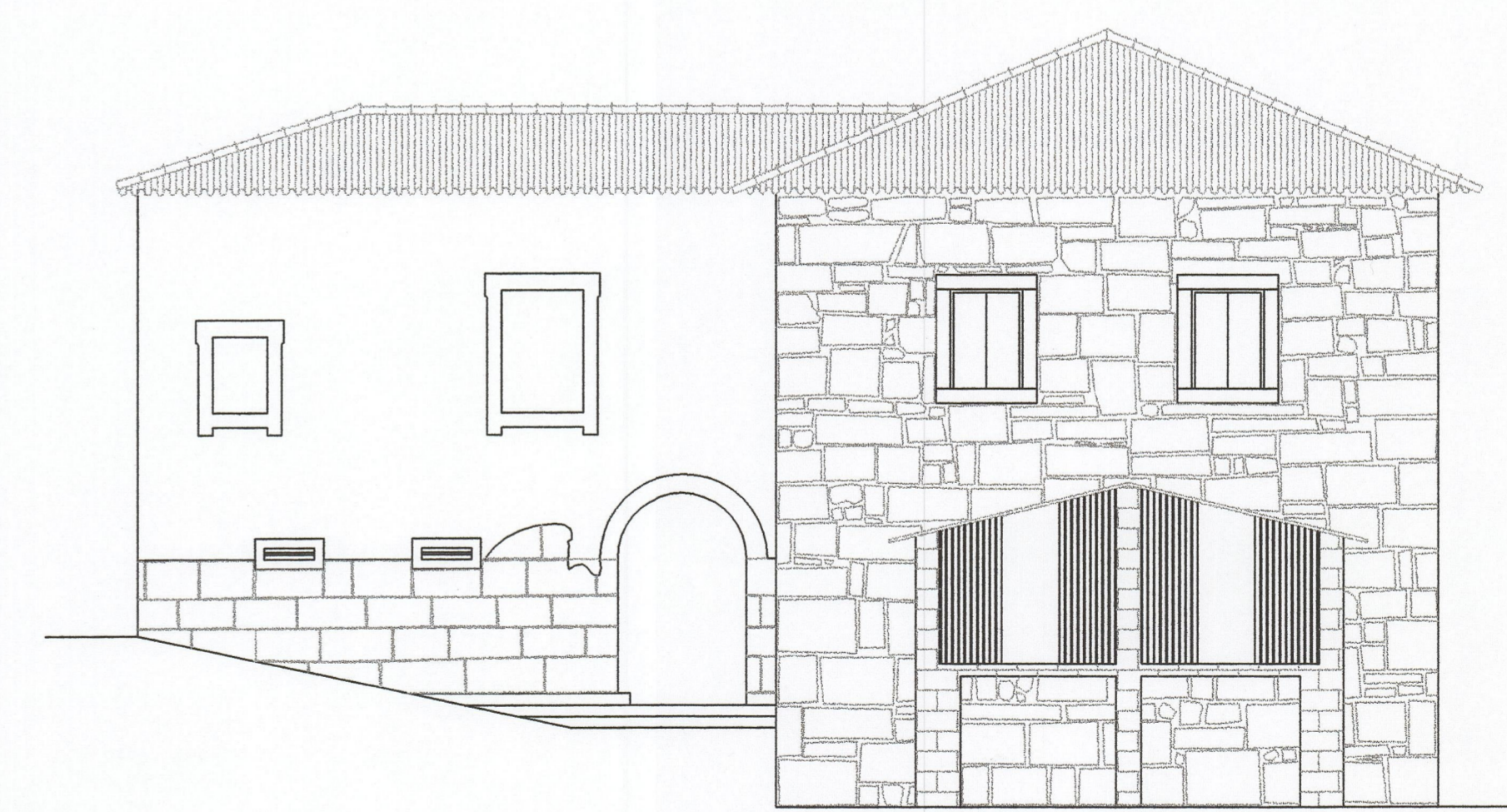
ALÇADO LAT. DIREITO
