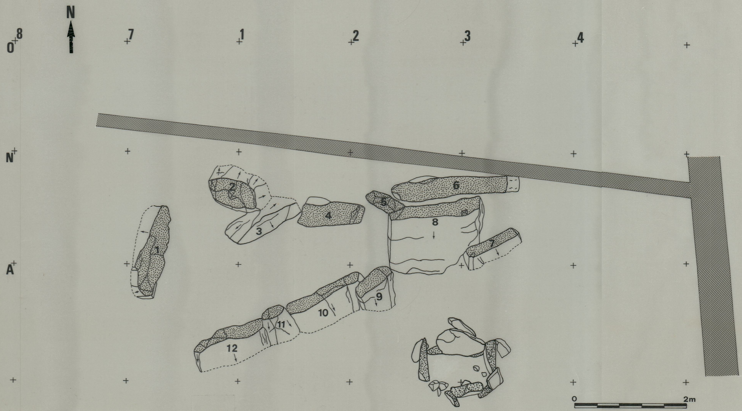
MAMOA DE S. ROMÃO DO NEIVA CASTELO DO NEIVA Planta da estrutura dolménica e cista
