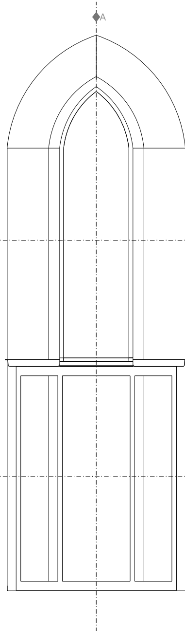
ALÇADO EXTERIOR
