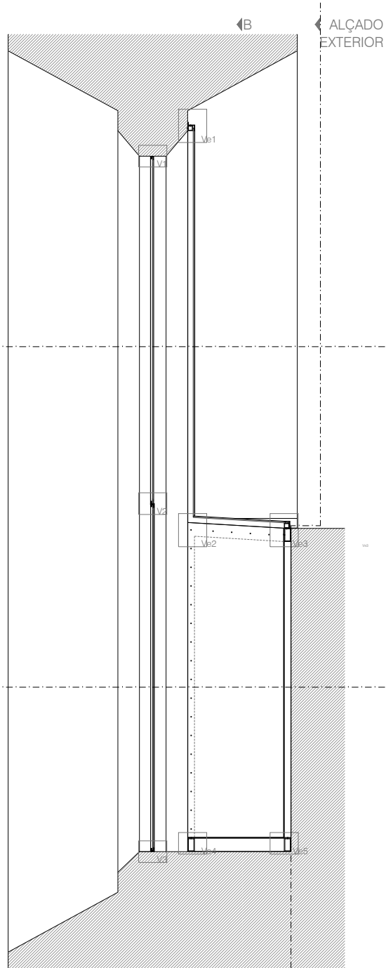
CORTE A
