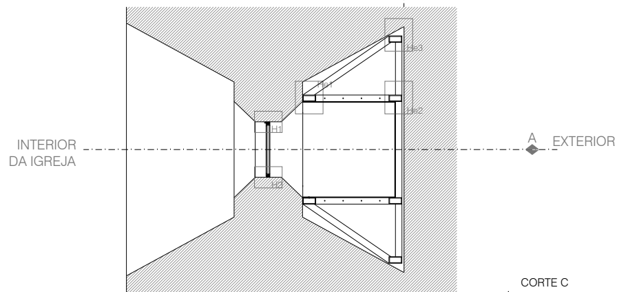
CORTE C
