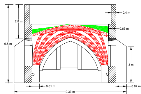
Corte 3-3
