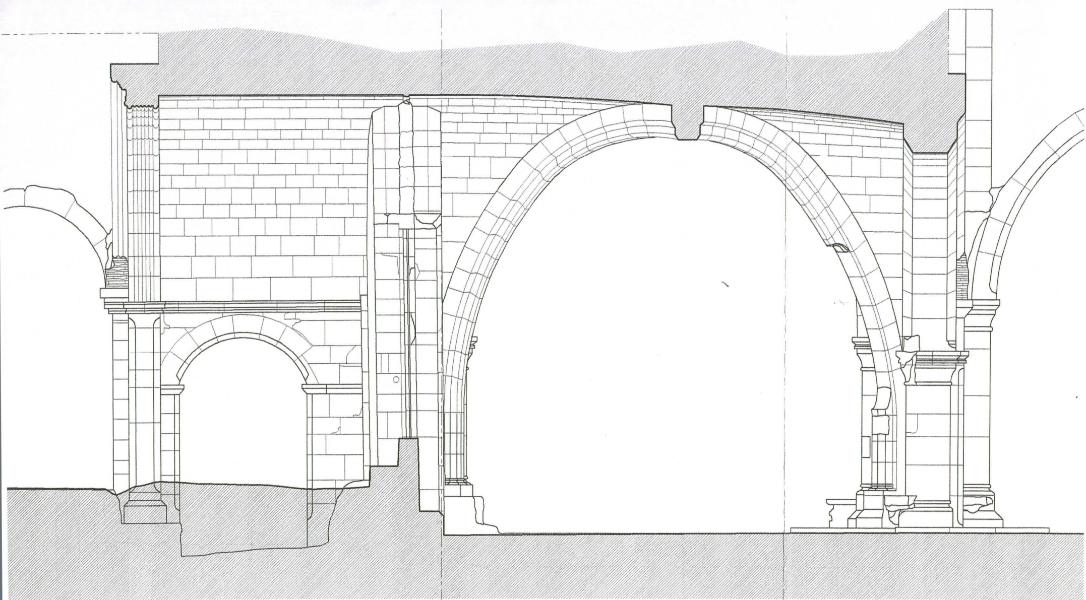
CORTE PELO EIXO DA IGREJA (junto à parede divisória) esc. 1/50
