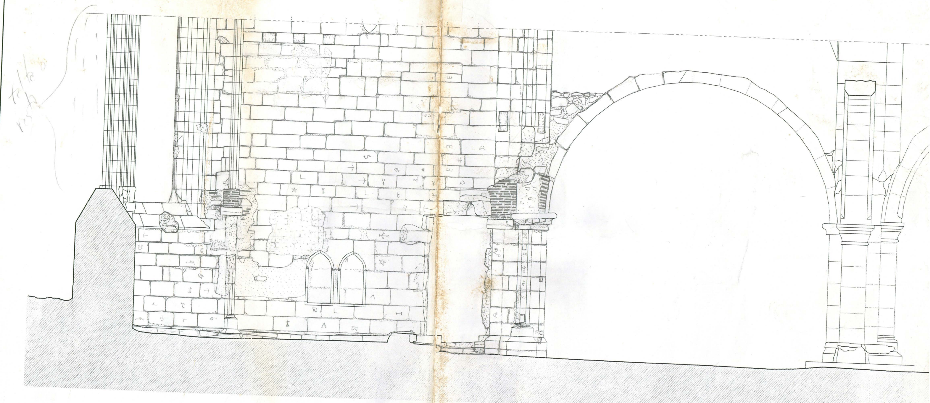
CORTE LONGITUDINAL 3b-3b'
