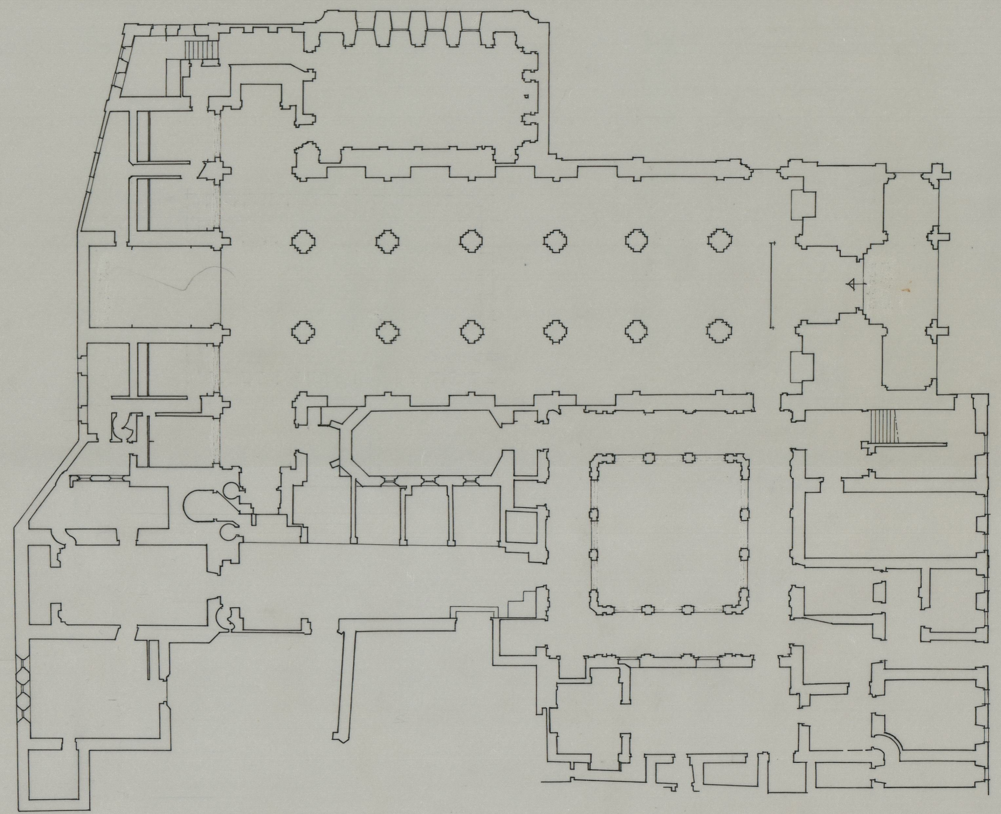
SÉ CATEDRAL DE BRAGA PLANTA GERAL
