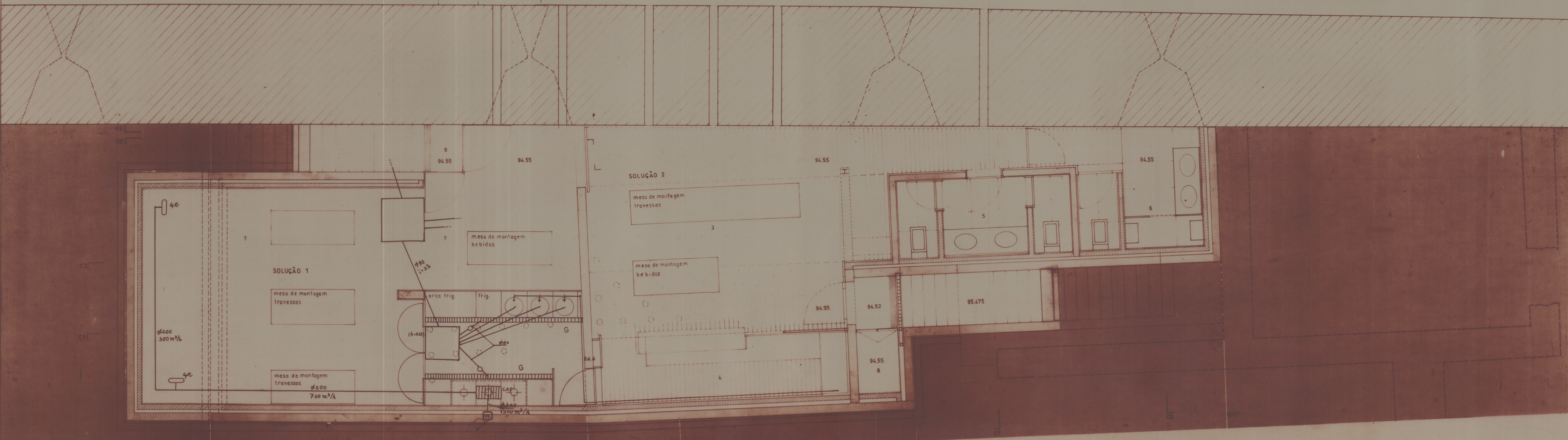
PLANTA À COTA 94.55
