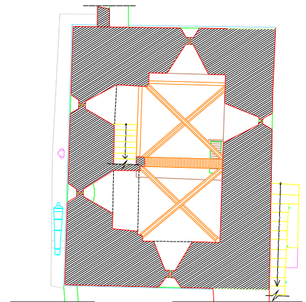
Planta Abóvadas Intermedia
