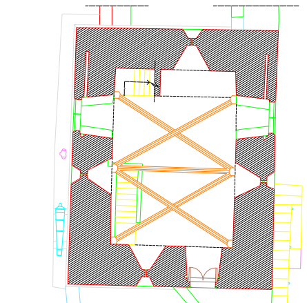
Planta Abóvadas Passagem da Ronda
