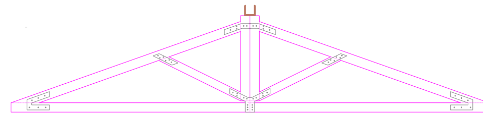
ASNA TIPO 1 1/20
