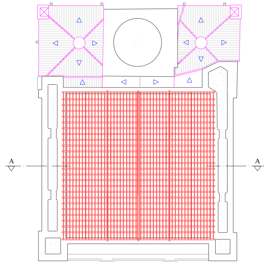
PLANTA DE ESTRUTURAS DA COBERTURA
