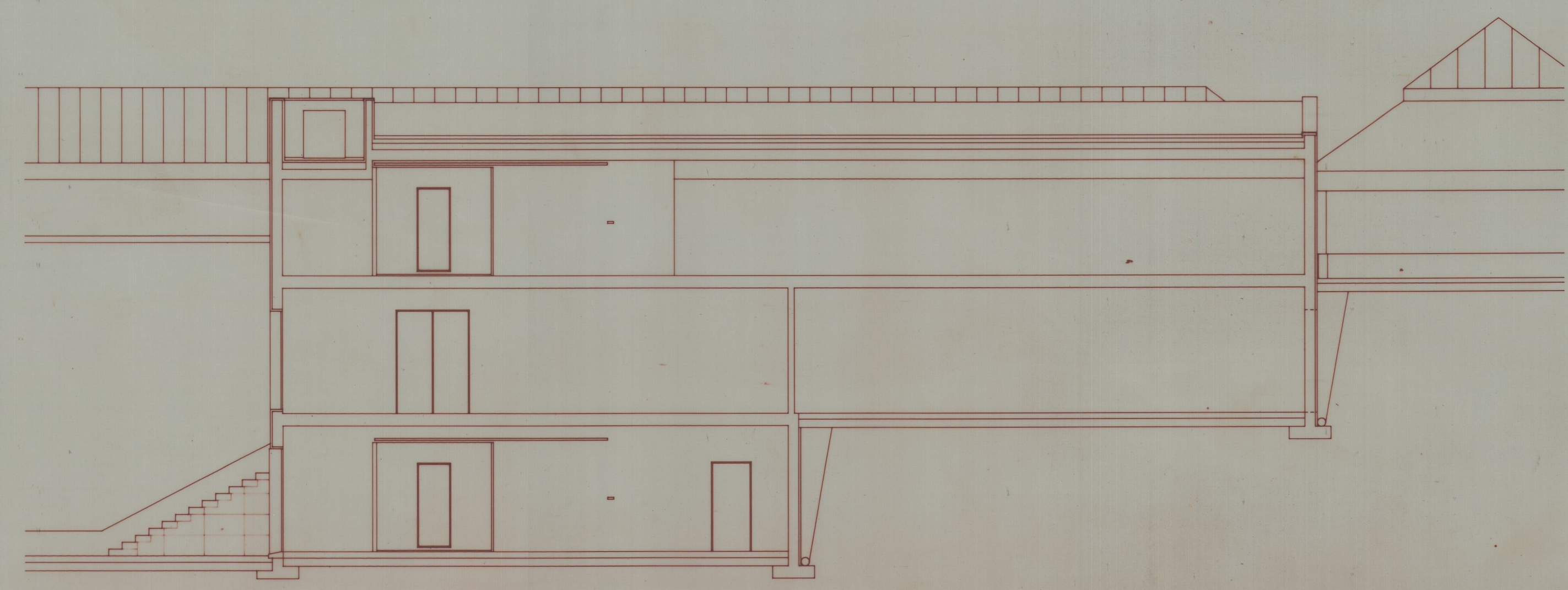
CORTE C4
