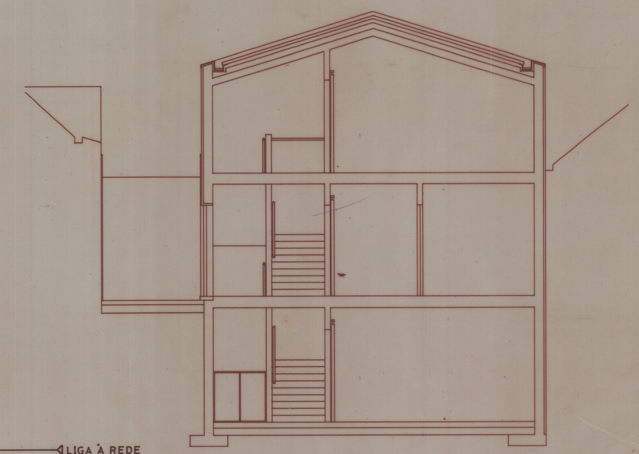
CORTE C1
