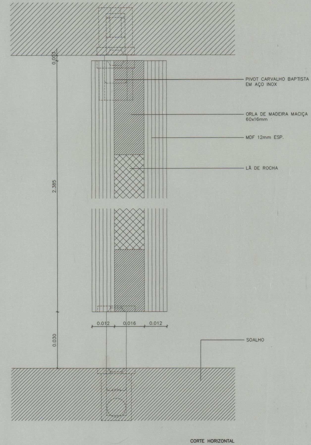
CORTE HORIZONTAL
