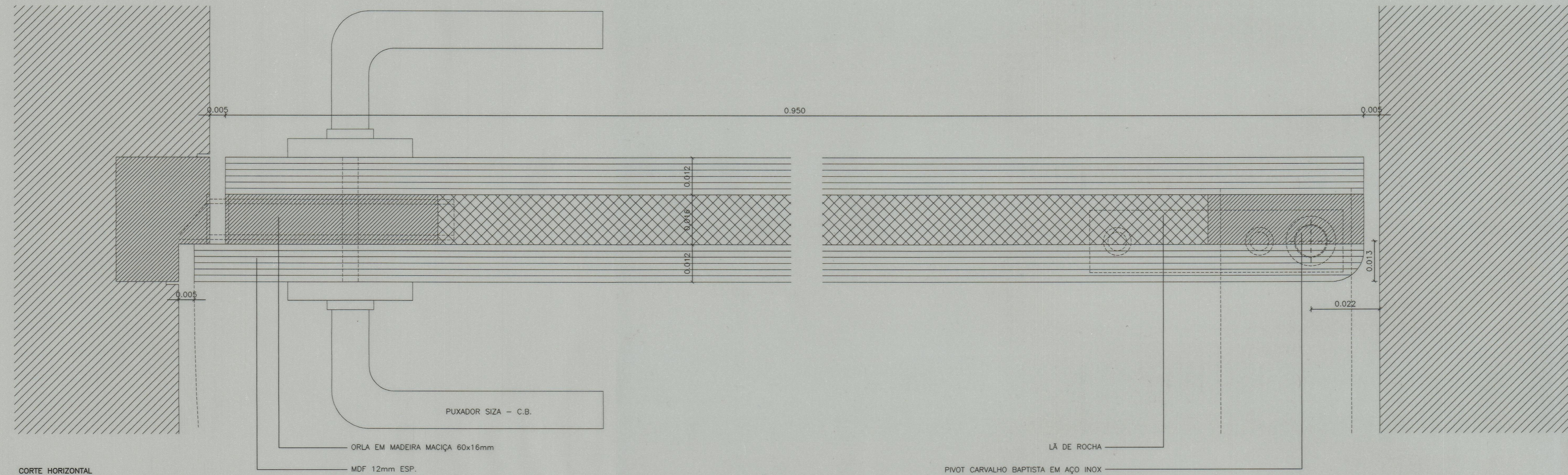
CORTE HORIZONTAL
