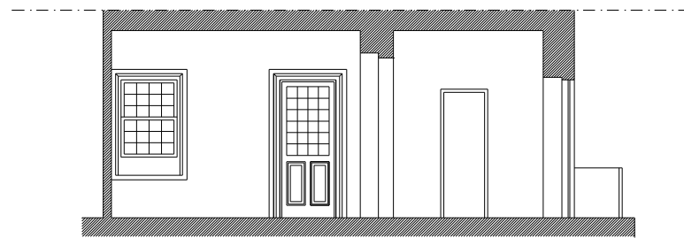
Corte A-A
