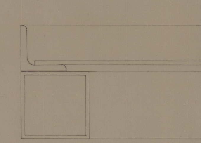
CORTE HORIZONTAL 1
