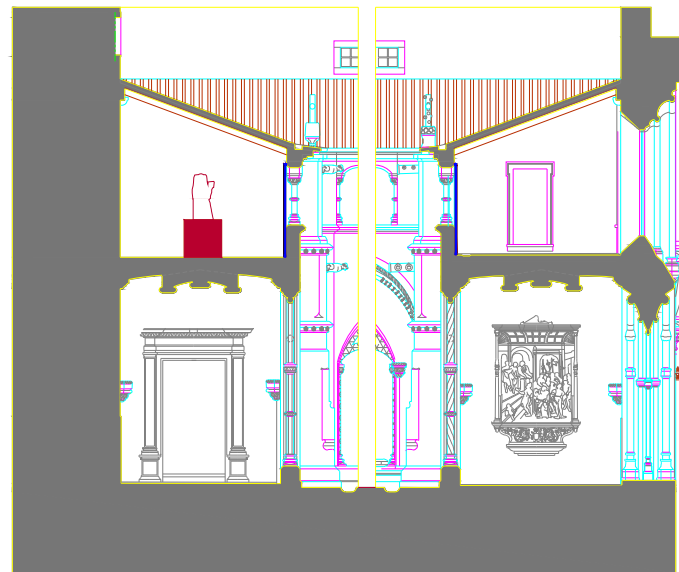
CORTE DA PROPOSTA
