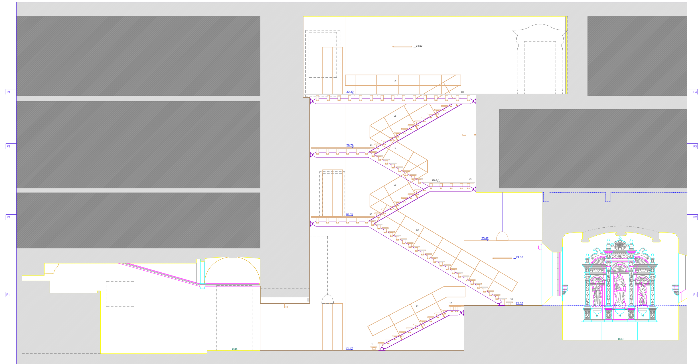
CORTE C1 - PROPOSTA
