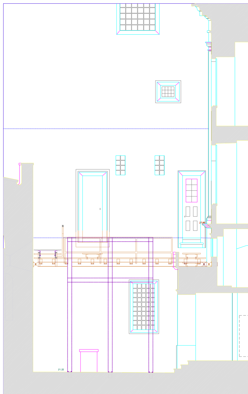
CORTE C1 - PROPOSTA
