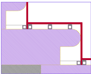
PORMENOR DA FORRA DAS ESCADAS
