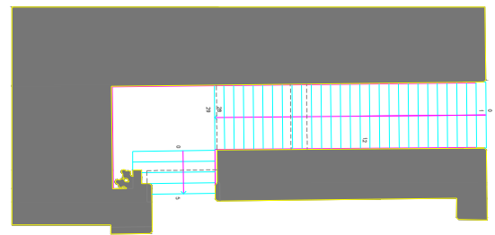
PLANTA DO EXISTENTE
