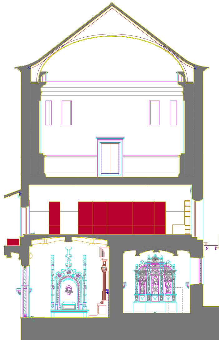
CORTE LONGITUDINAL DA PROPOSTA
