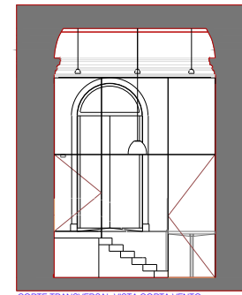
CORTE TRANSVERSAL-VISTA CORTA VENTO
