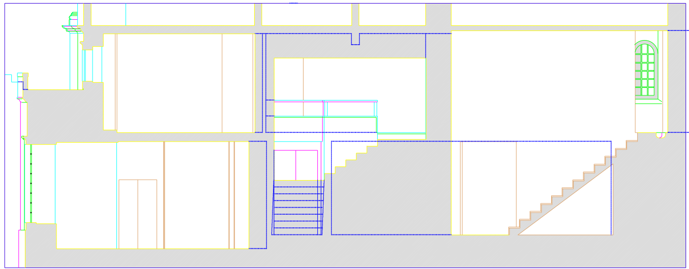
CORTE C1 - PROPOSTA
