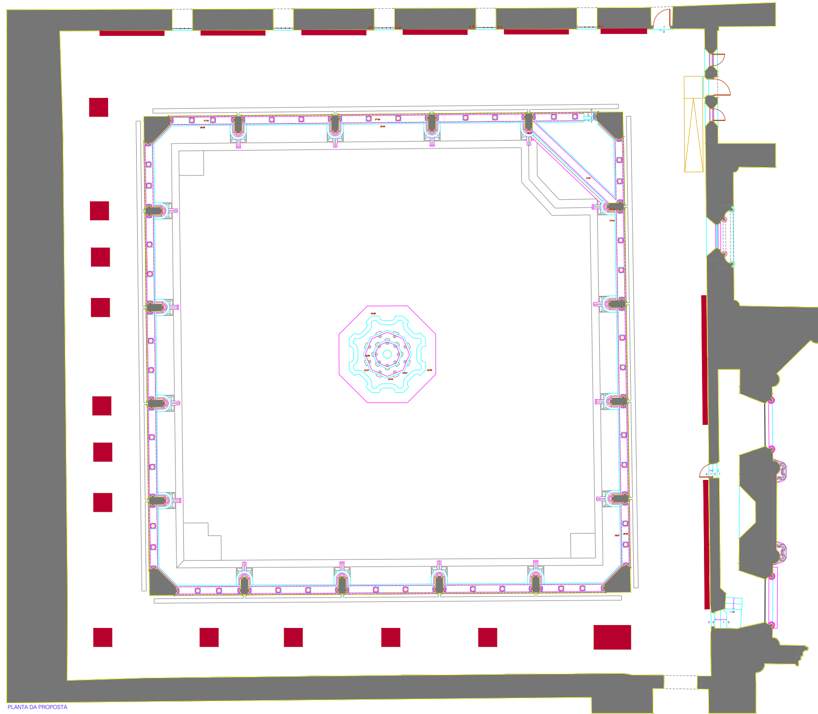
PLANTA DA PROPOSTA
