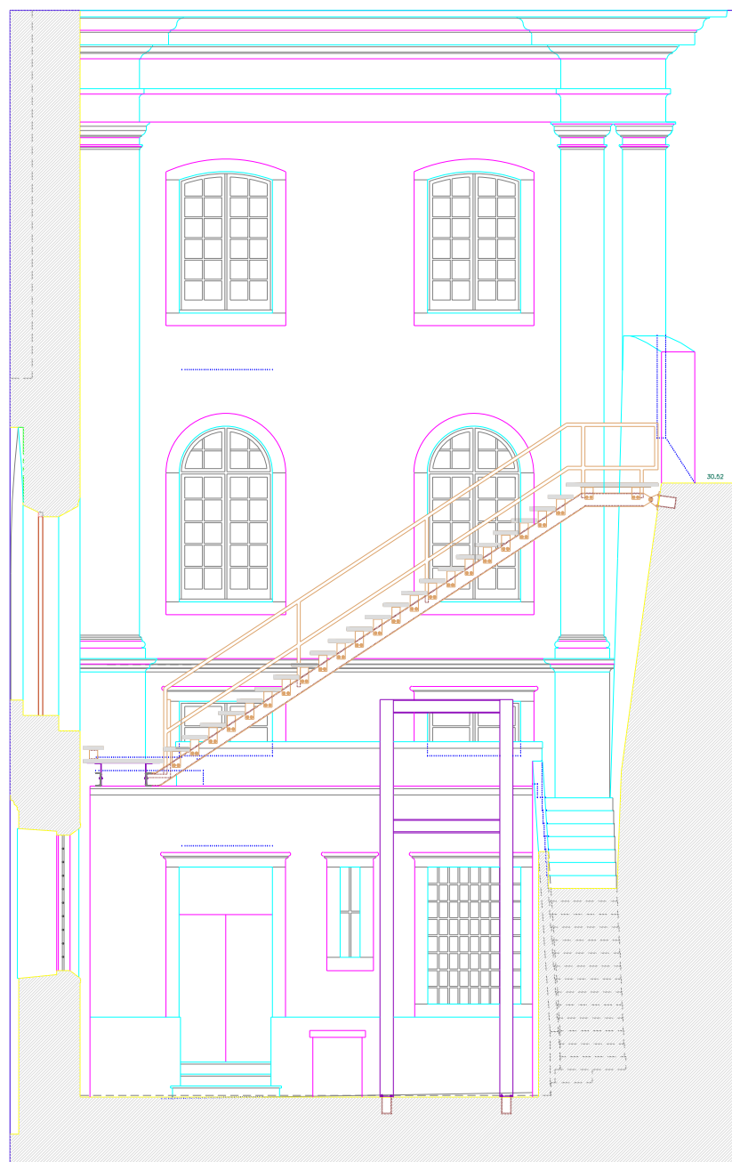
CORTE C2 - PROPOSTA
