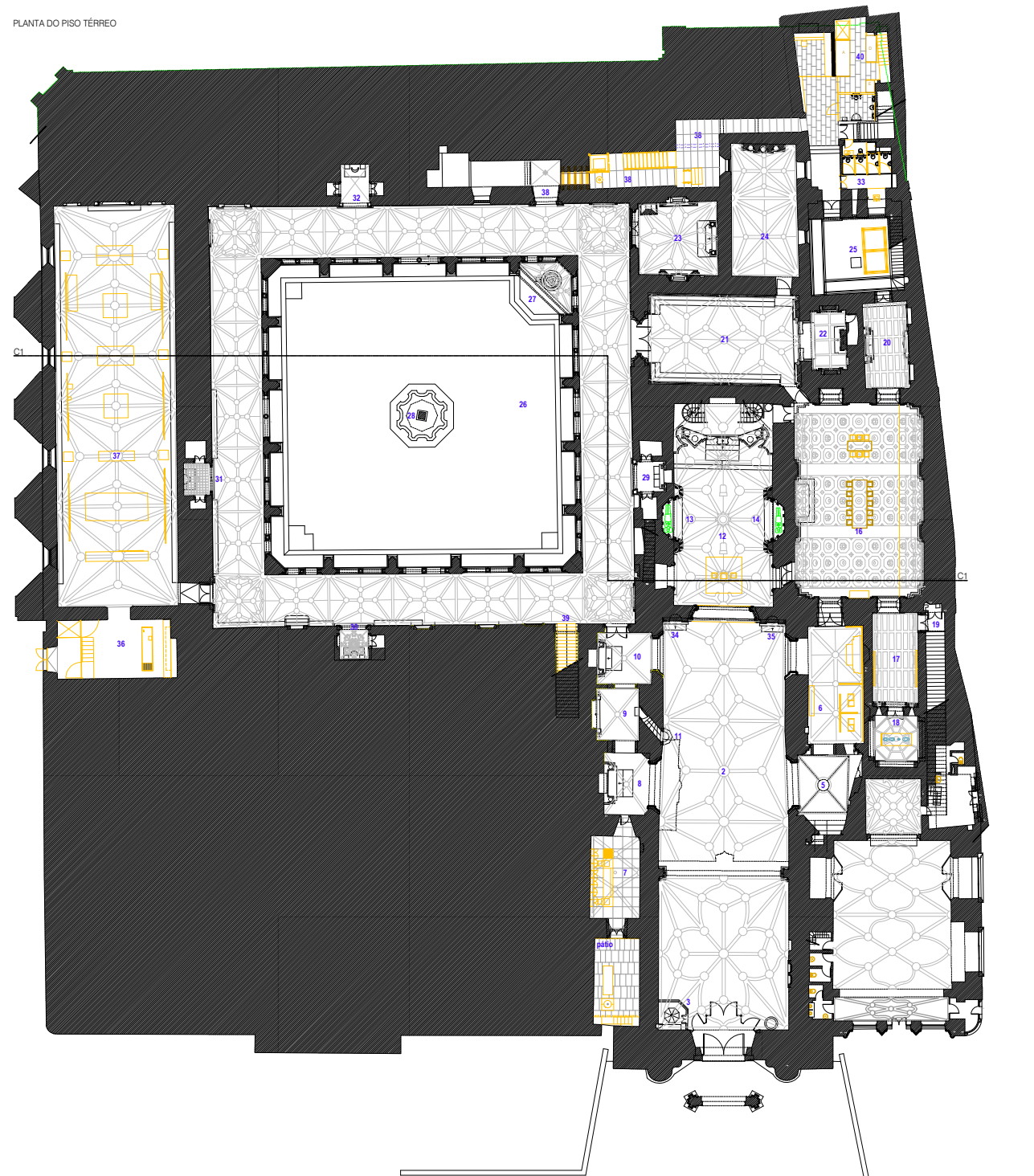
PLANTA DO 1º PISO (SOBRECLAUSTRO)
