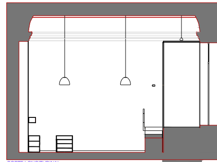
CORTE LONGITUDINAL
