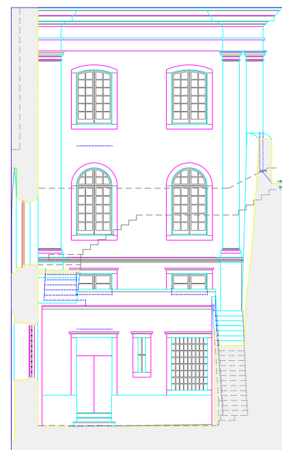
CORTE C2 - EXISTENTE
