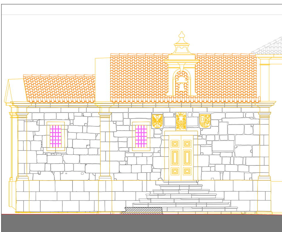
ALÇADO OESTE ANTES DA INTERVENÇÃO
