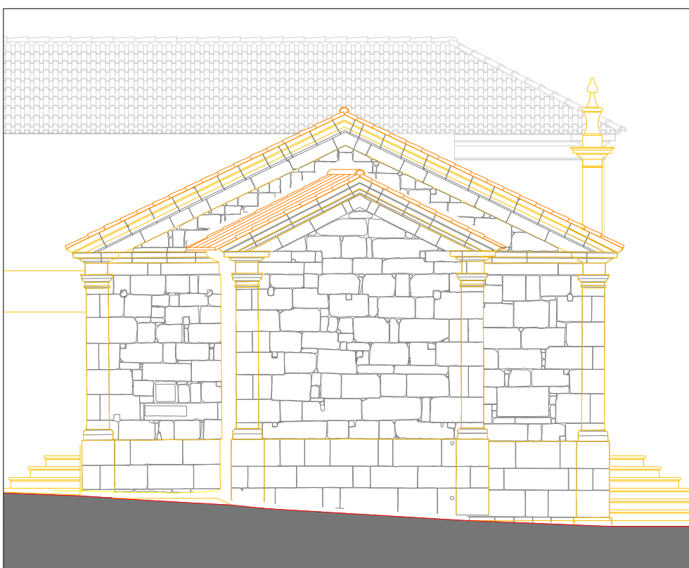
ALÇADO NORTE ANTES DA INTERVENÇÃO
