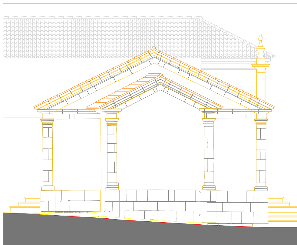
ALÇADO NORTE DEPOIS DA INTERVENÇÃO
