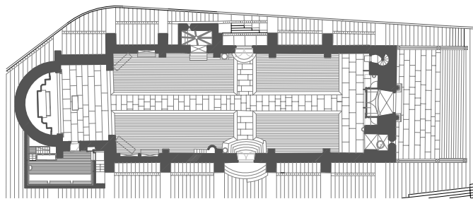
Planta do piso térreo
