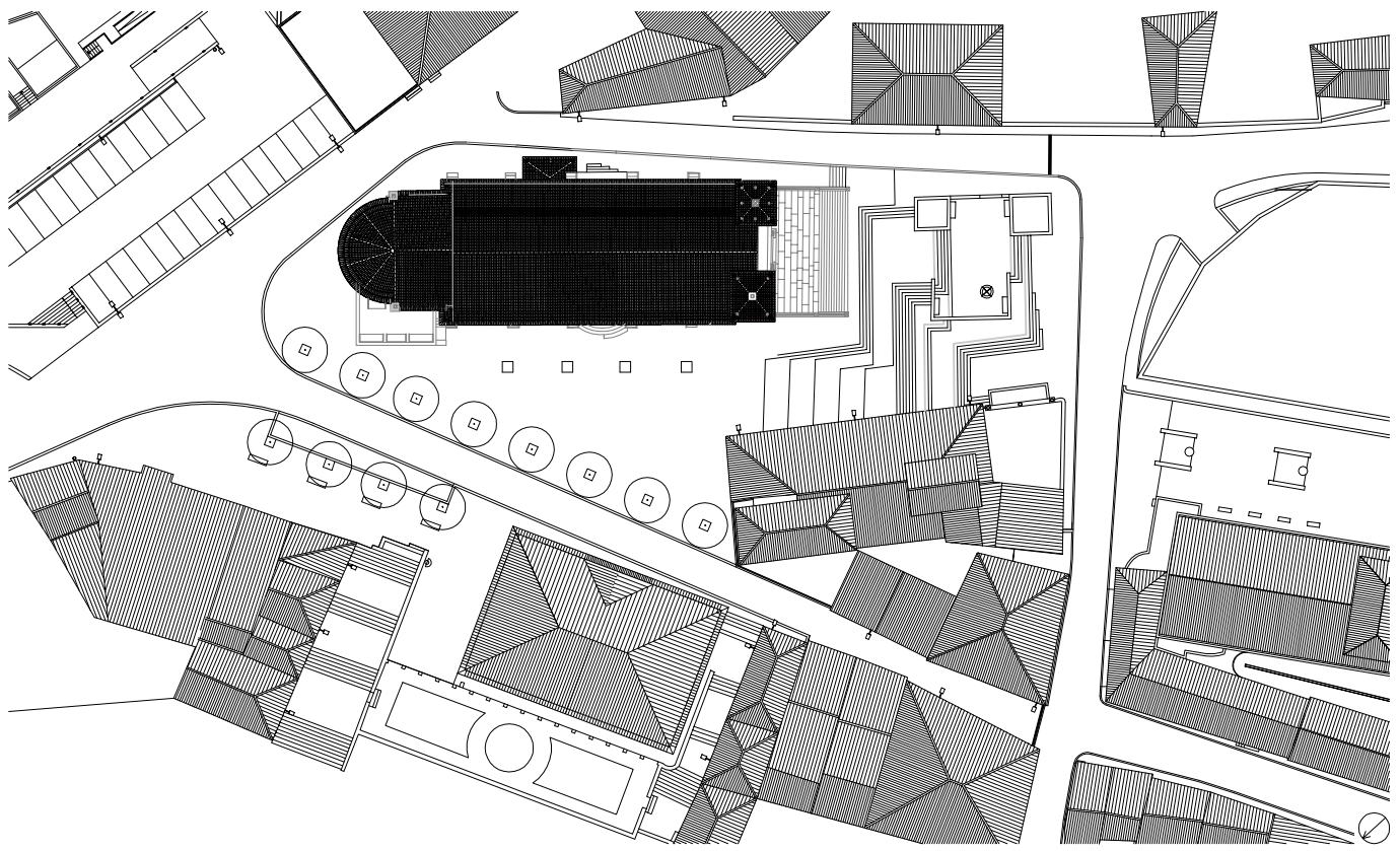
Implantação
