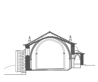
Corte transversal
