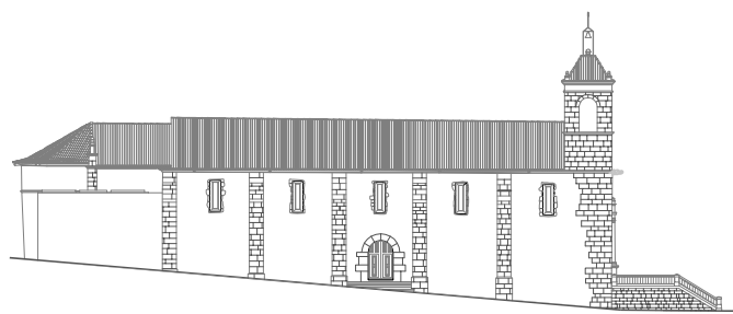
Alçado noroeste
