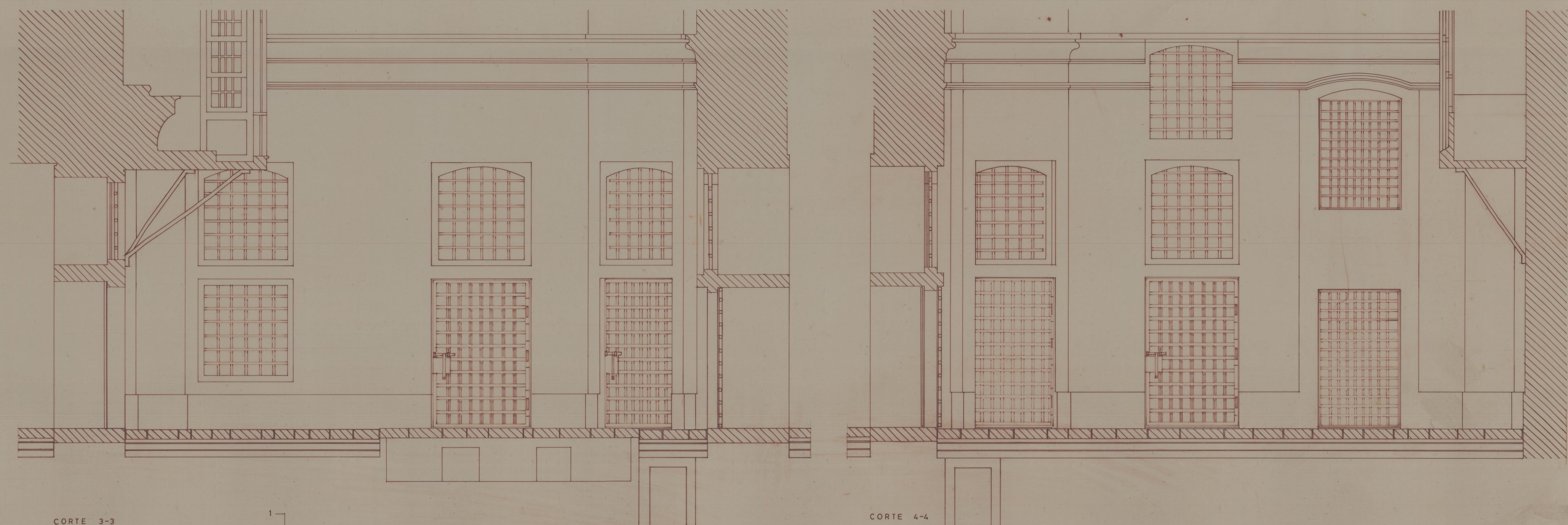
CORTE 3-3
