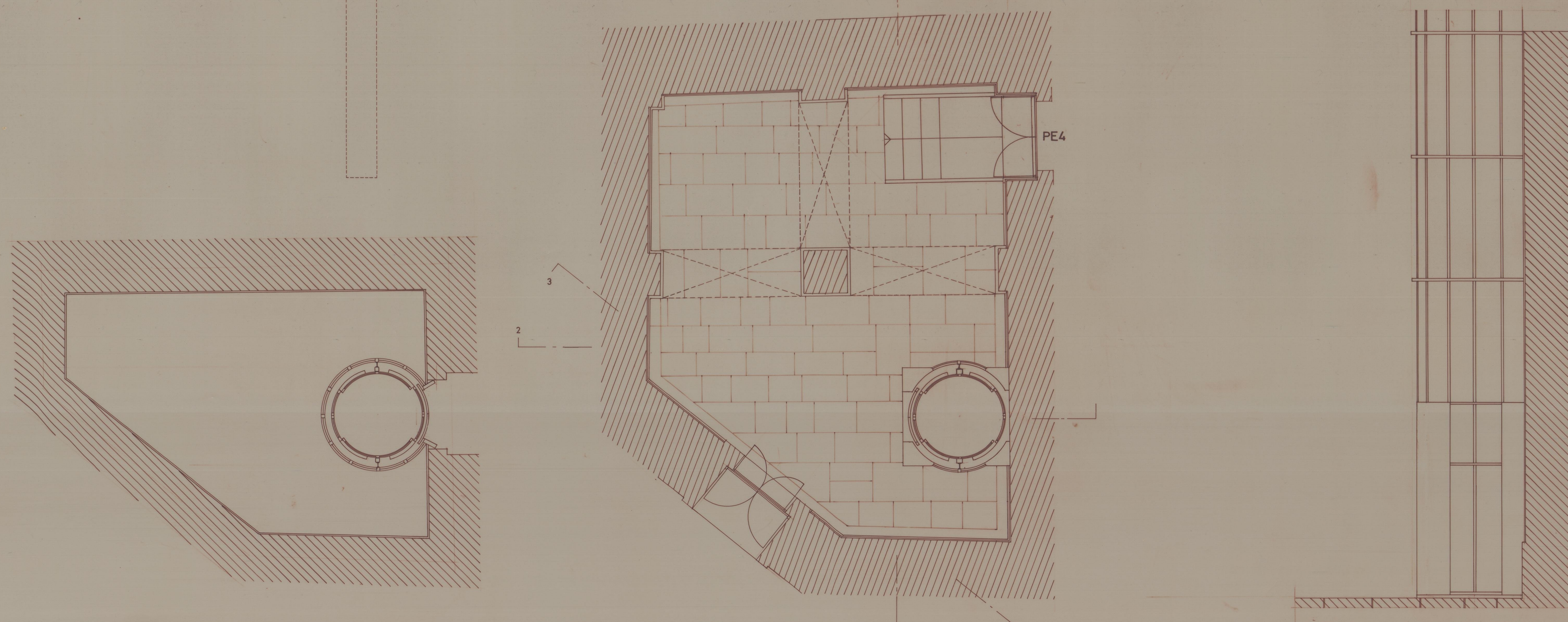
PLANTA DO SAGUZO
