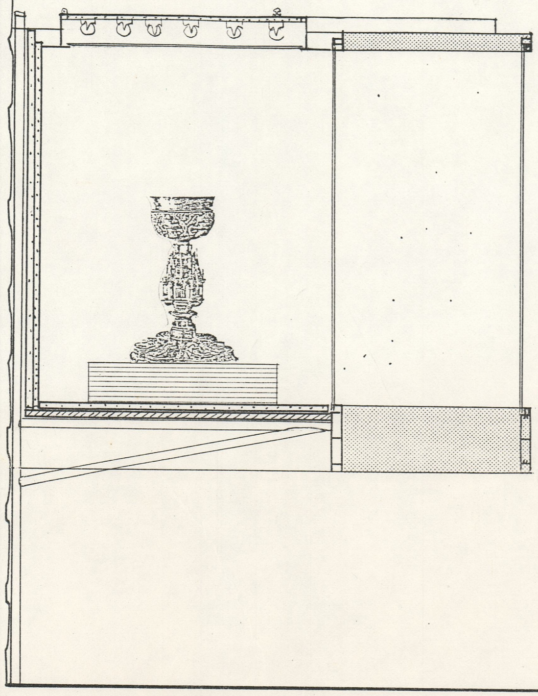
CORTE ESC 1/10
