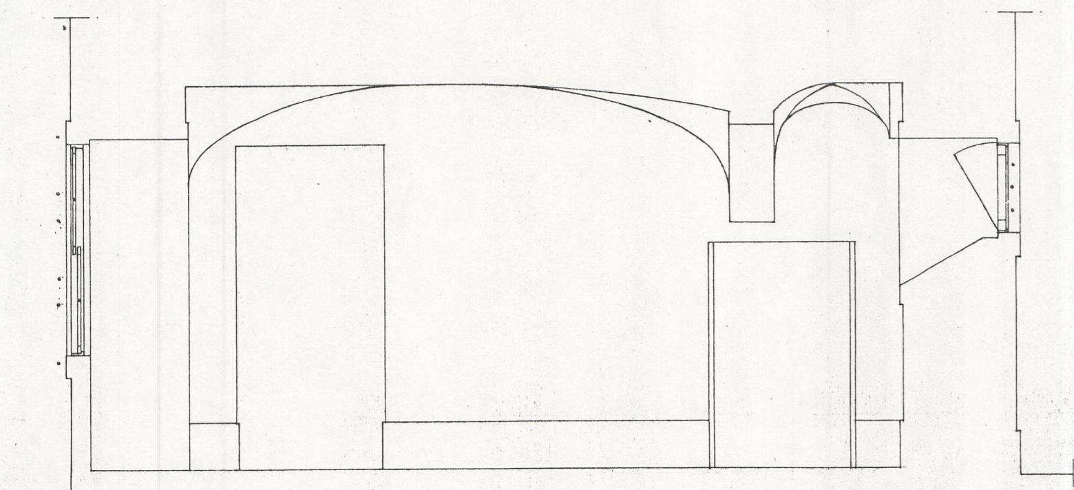
CORTE C3
