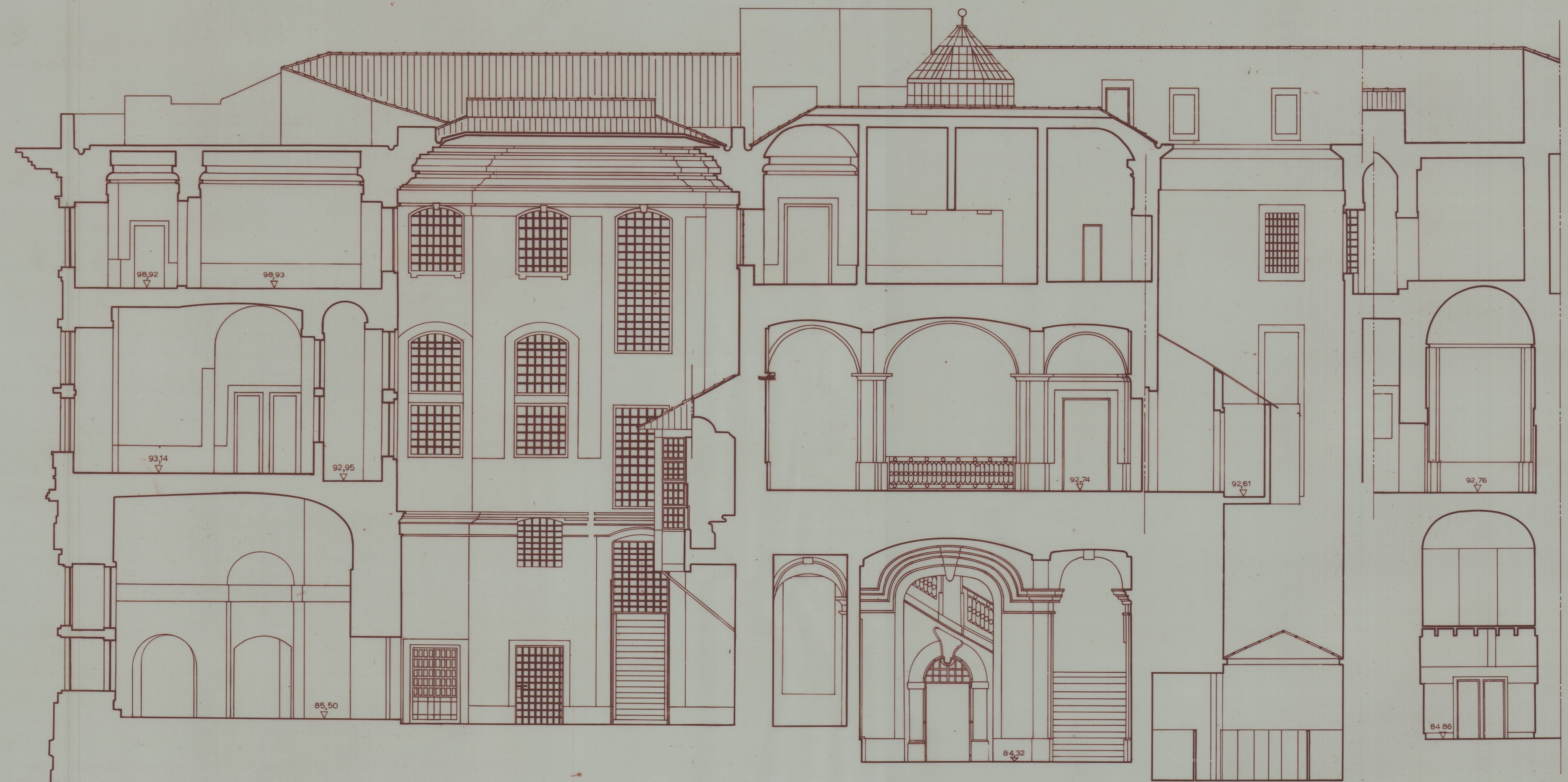
CORTE D-D
