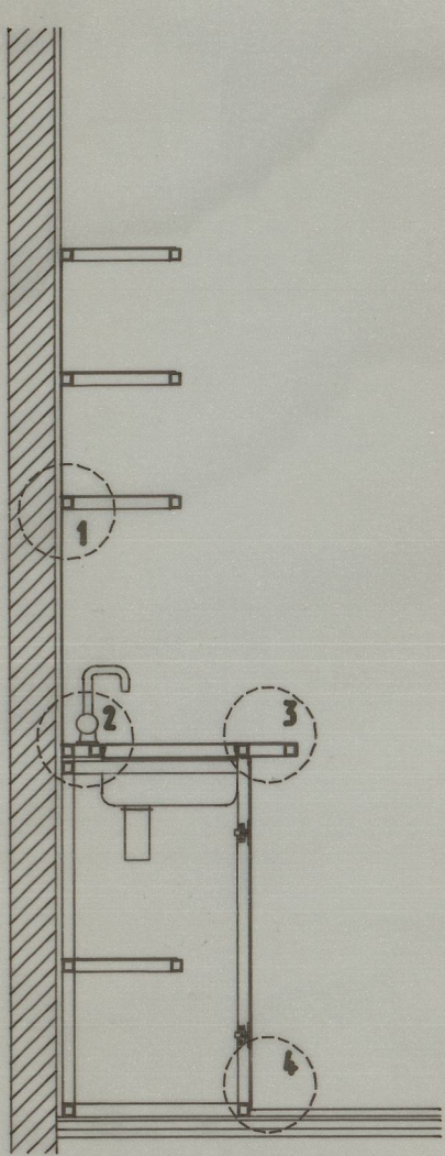
CORTE 2.2
