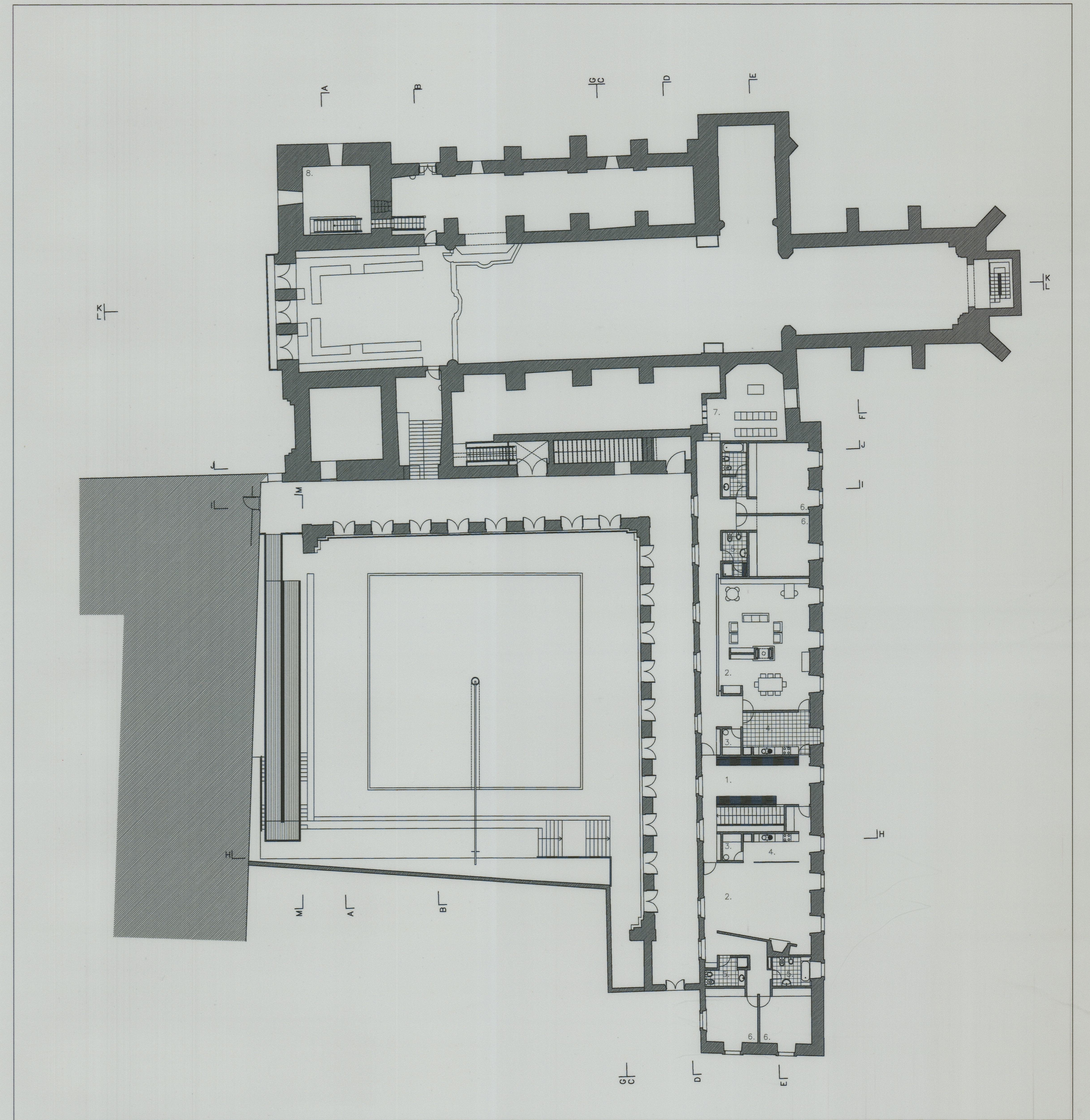
PLANTA DO PISO 2. PROPOSTO LEGENDA: 1. VESTIBULO 2. SALA COMUM 3. DESPENSA 4. COZINHA 5. CASA DE BANHO 6. QUARTO 7. CAPELA DO NOVOÇAO 8. ESCADA DE ACESSO ATORRE
