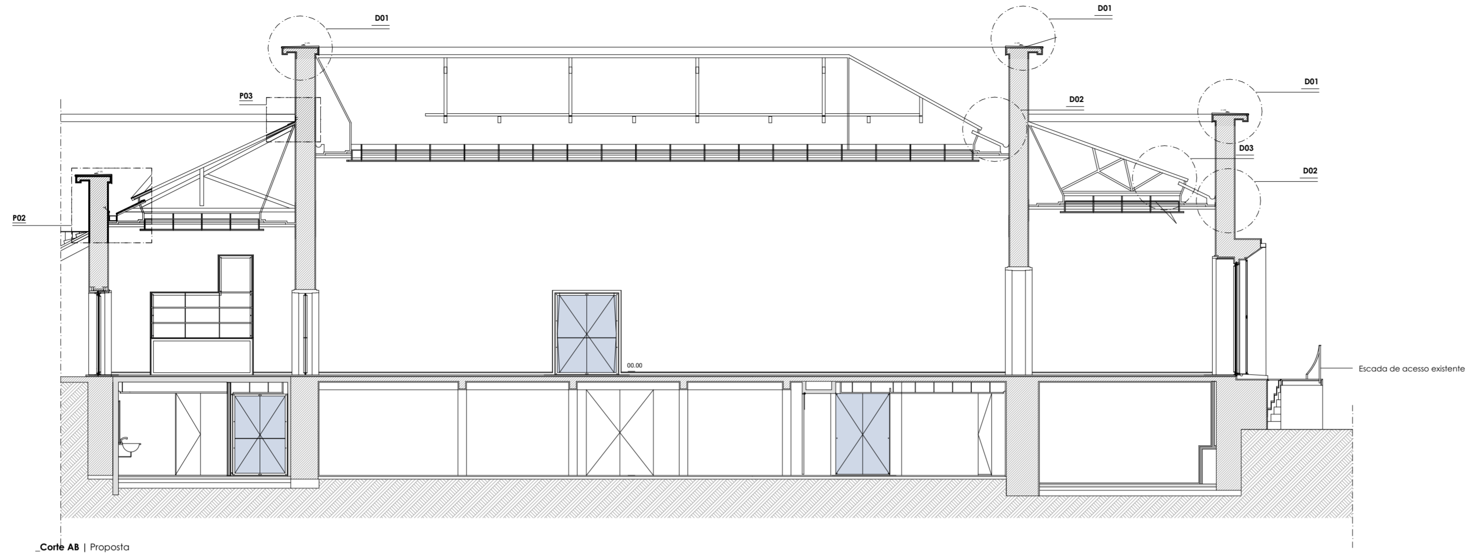
_Corte AB | Proposta
