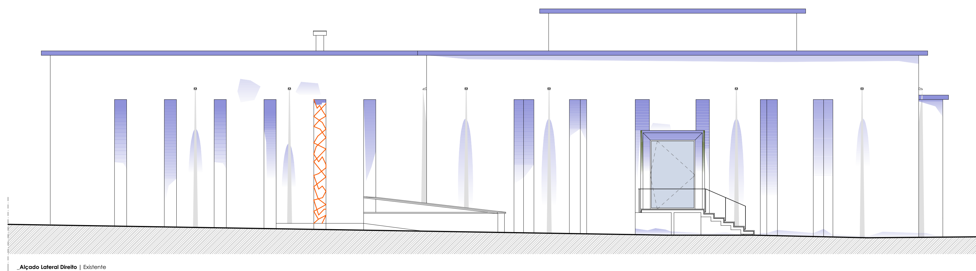
Alçado Lateral Direito | Existente
