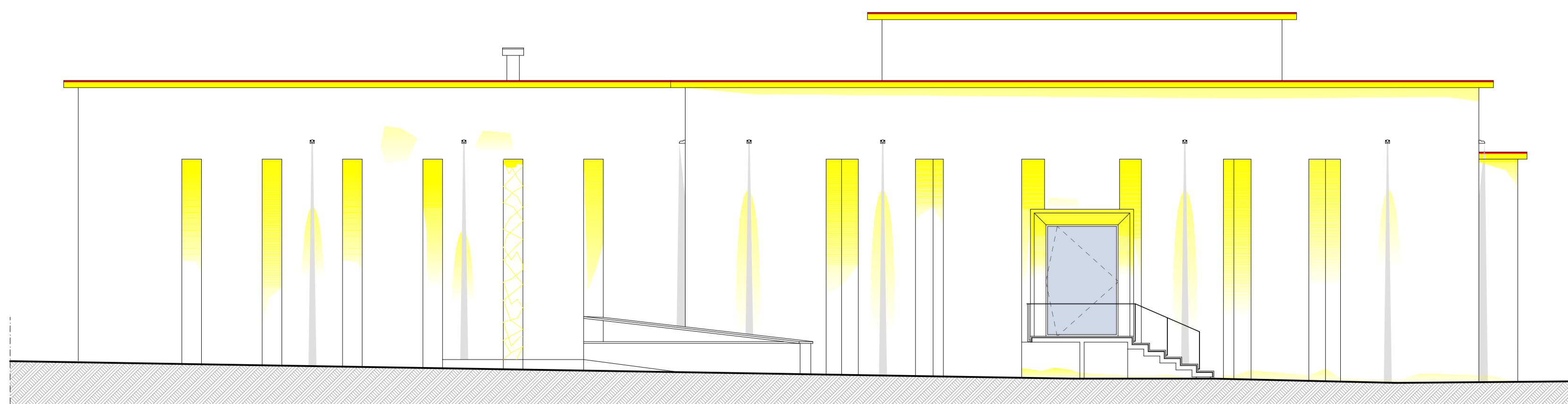
Alçado Lateral Direito | AV - Alterações
