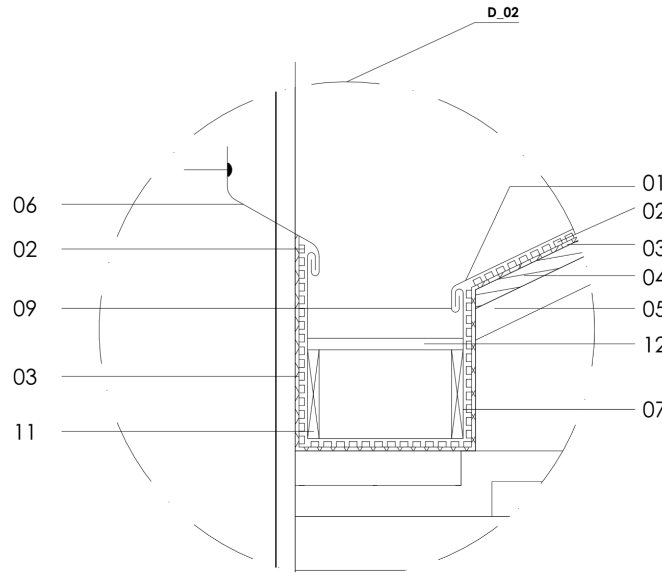
D_02 esc: 1/5
