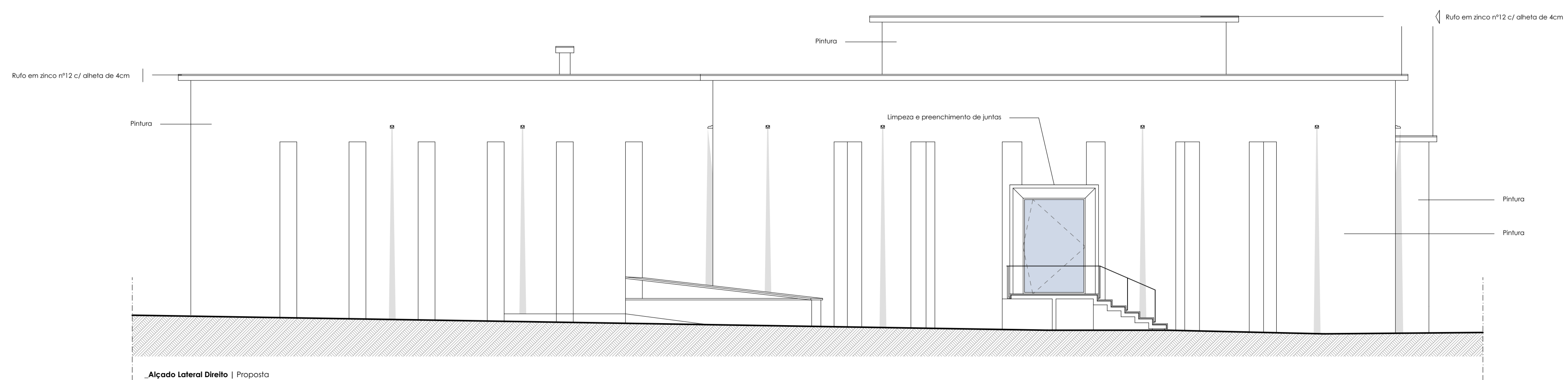
Alçado Lateral Direito | Proposta
