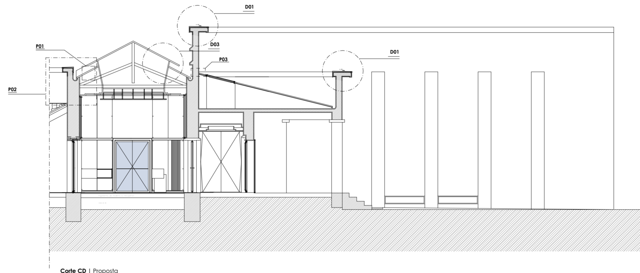
_Corte CD | Proposta
