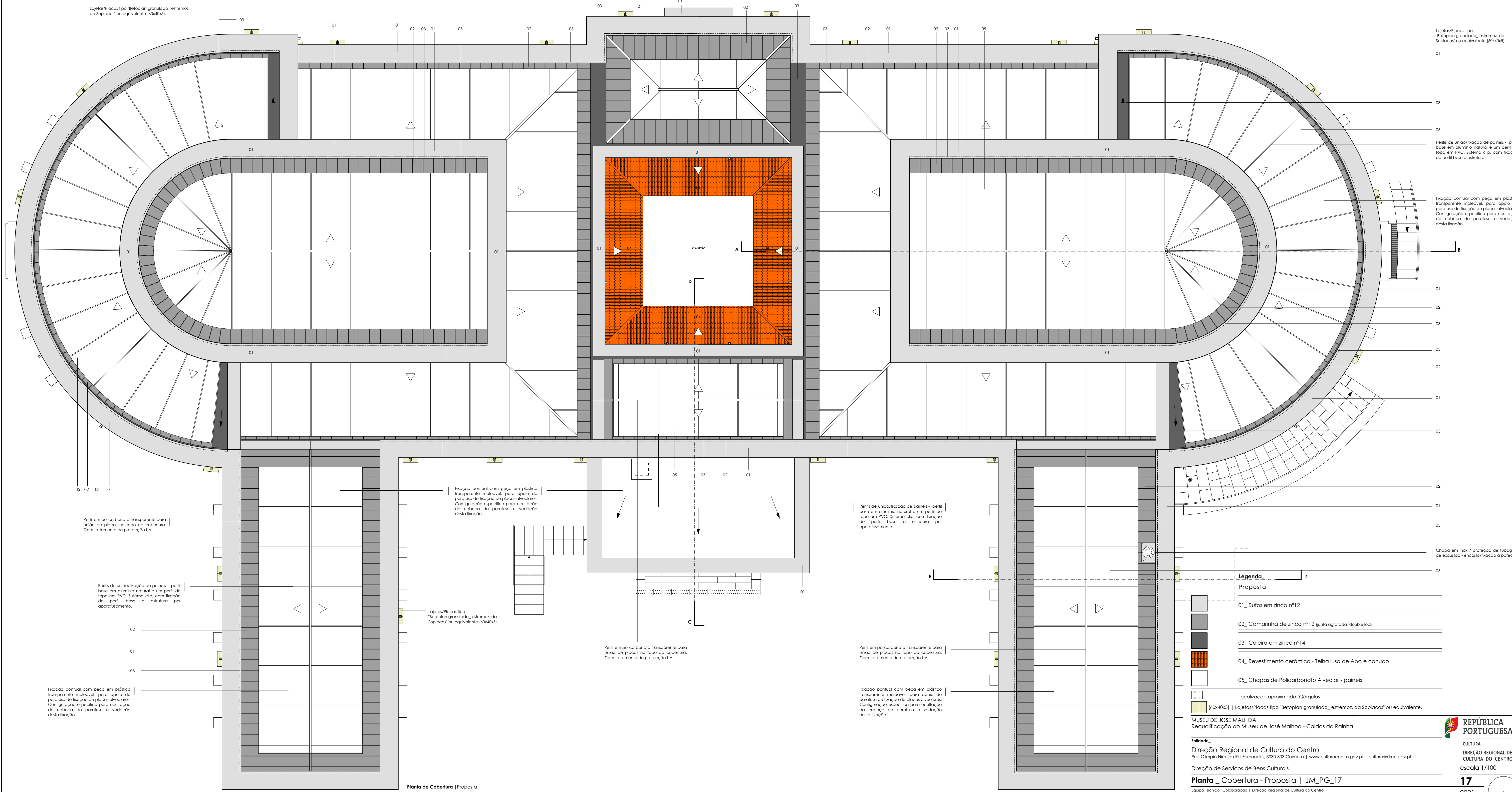
Planta de Cobertura | Proposta
