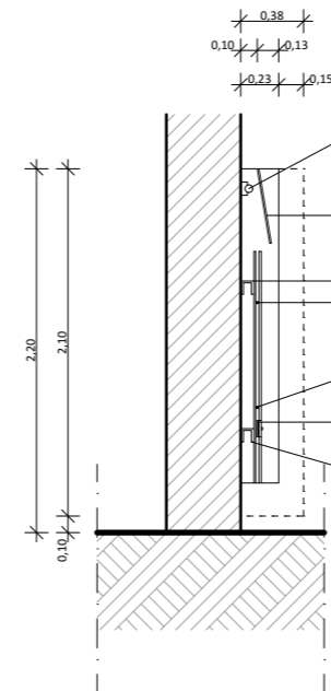
_Vista | Lateral/corte vertical (cv)
