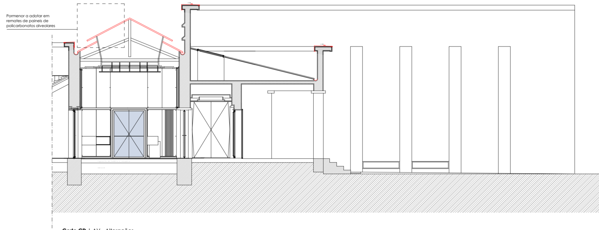
_Corte CD | AV - Alterações
