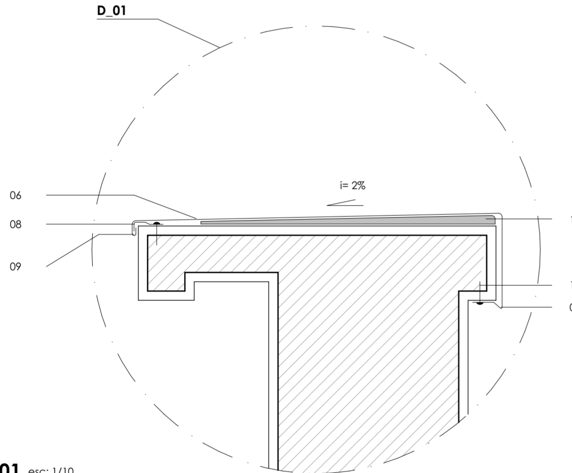
D_01 esc: 1/10
