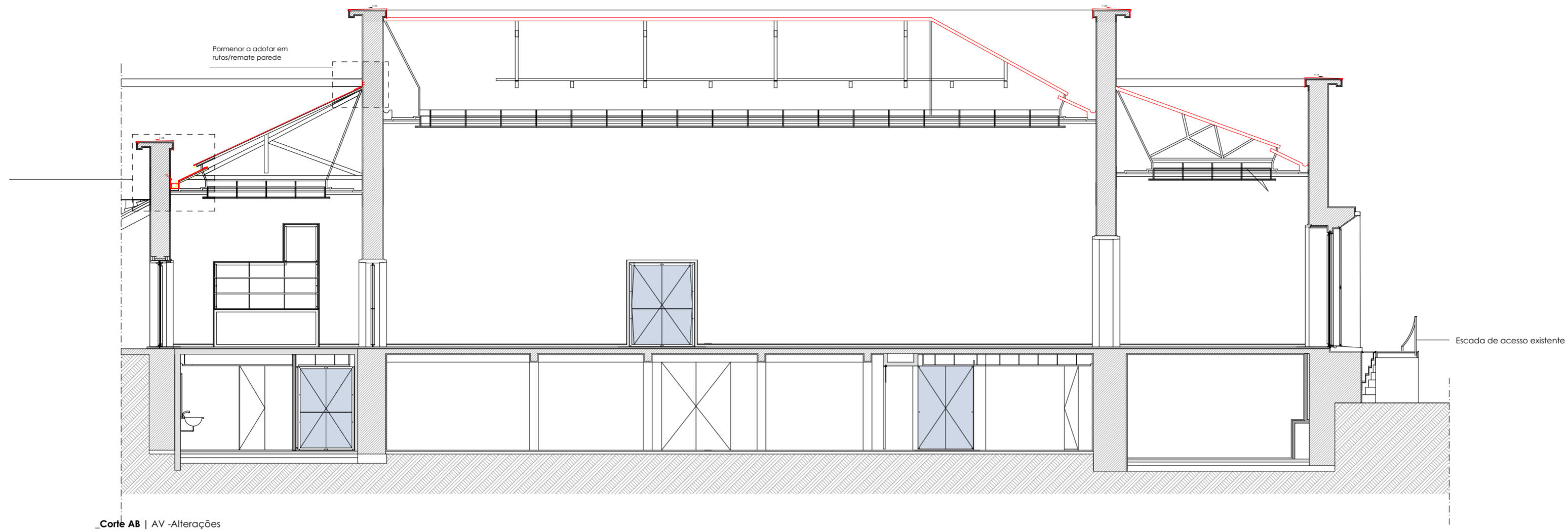
_Corte AB | AV - Alterações
