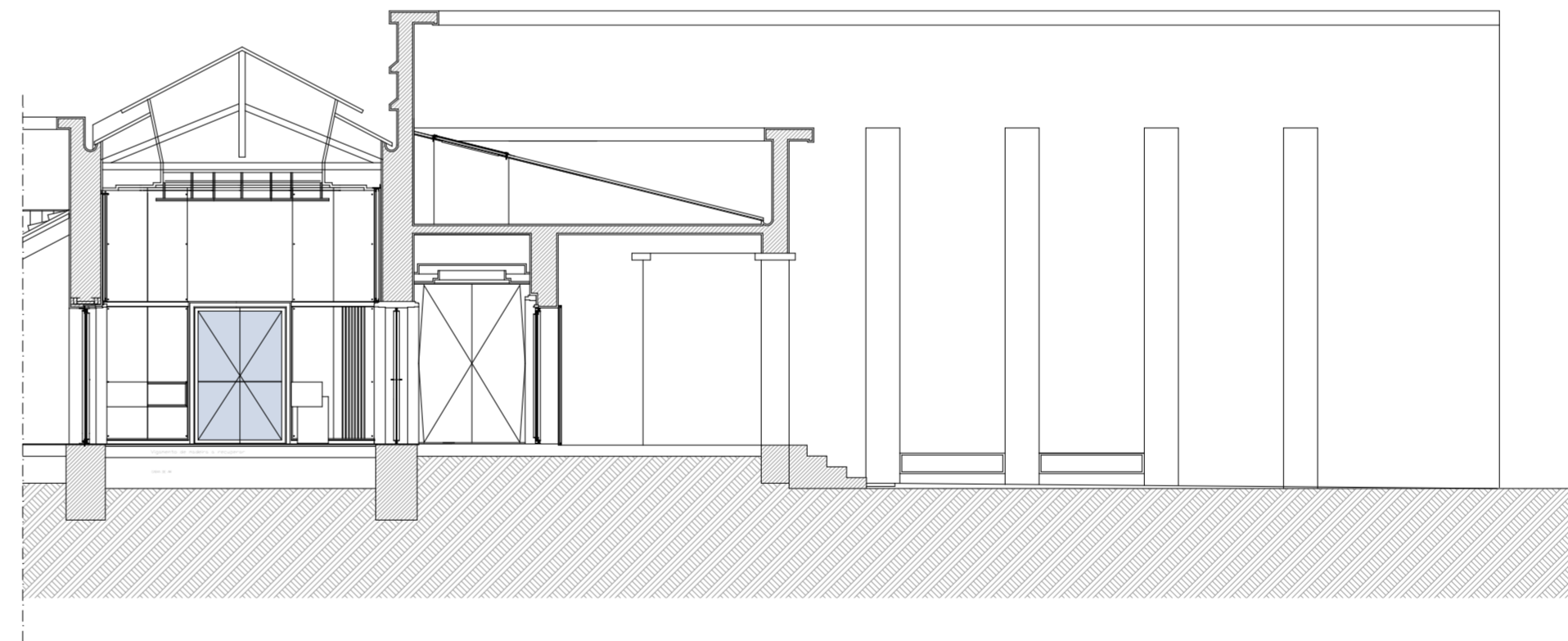
_Corte CD | Existente
