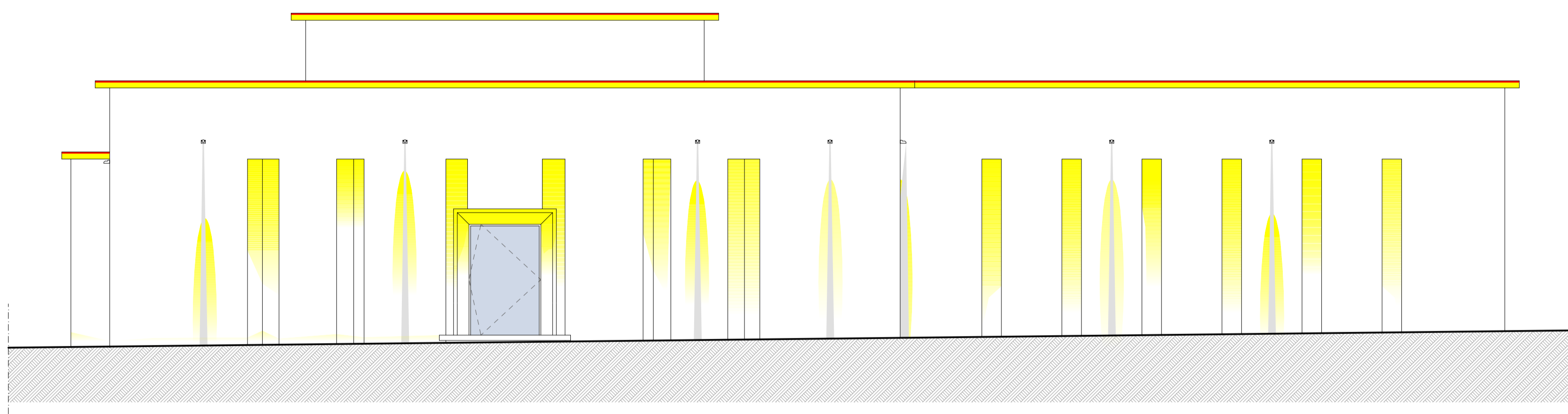
Alçado Lateral Esquerdo | AV - Alterações
