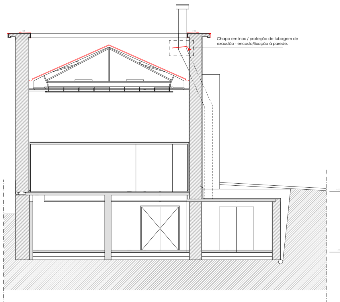
_Corte EF | AV - Alterações
