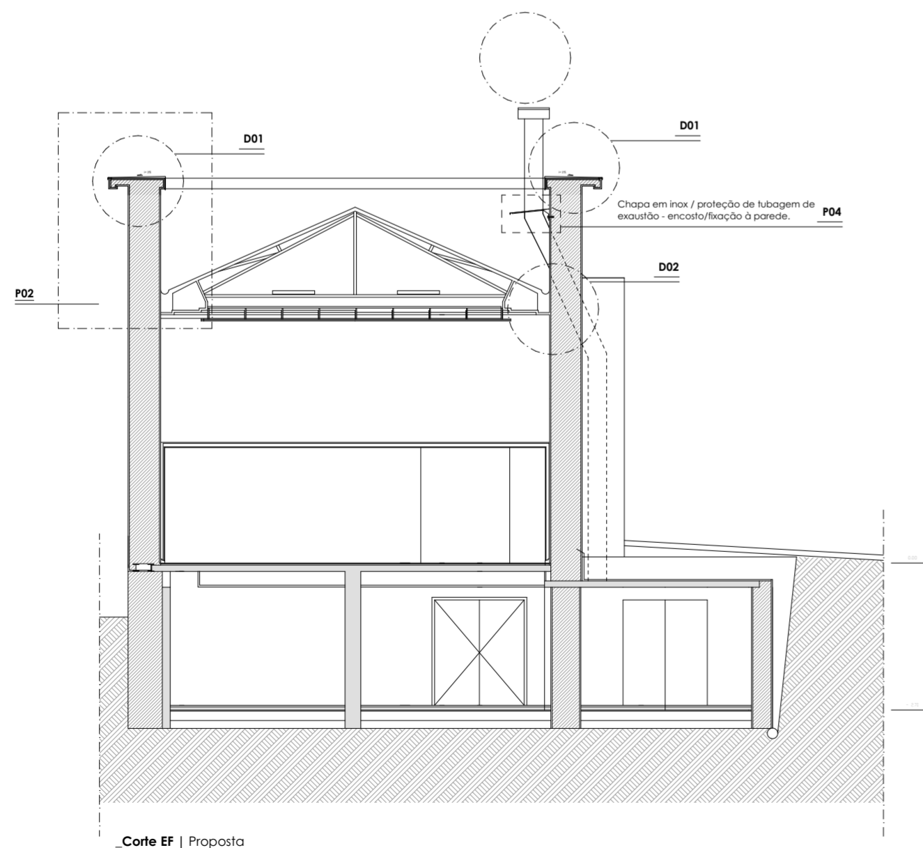
_Corte EF | Proposta
