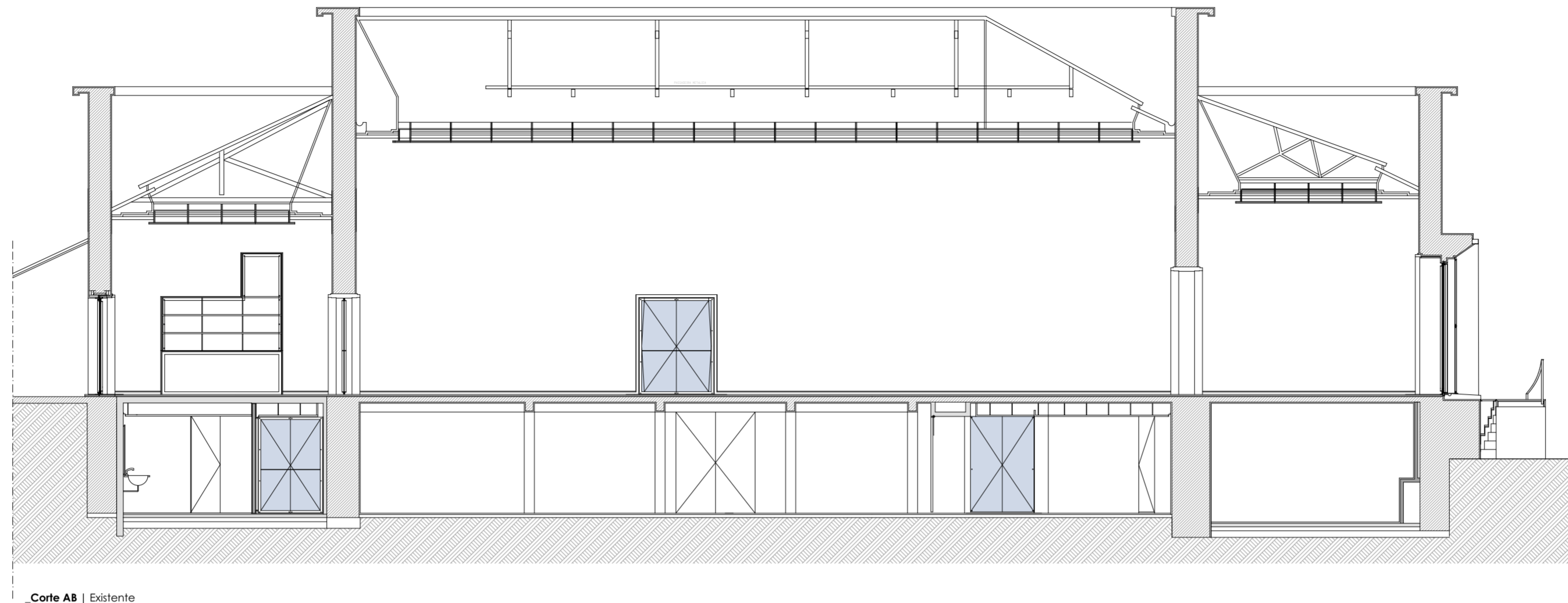
_Corte AB | Existente
