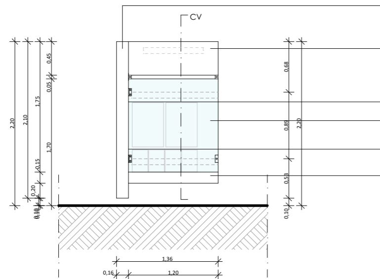
_Vista | Frente
