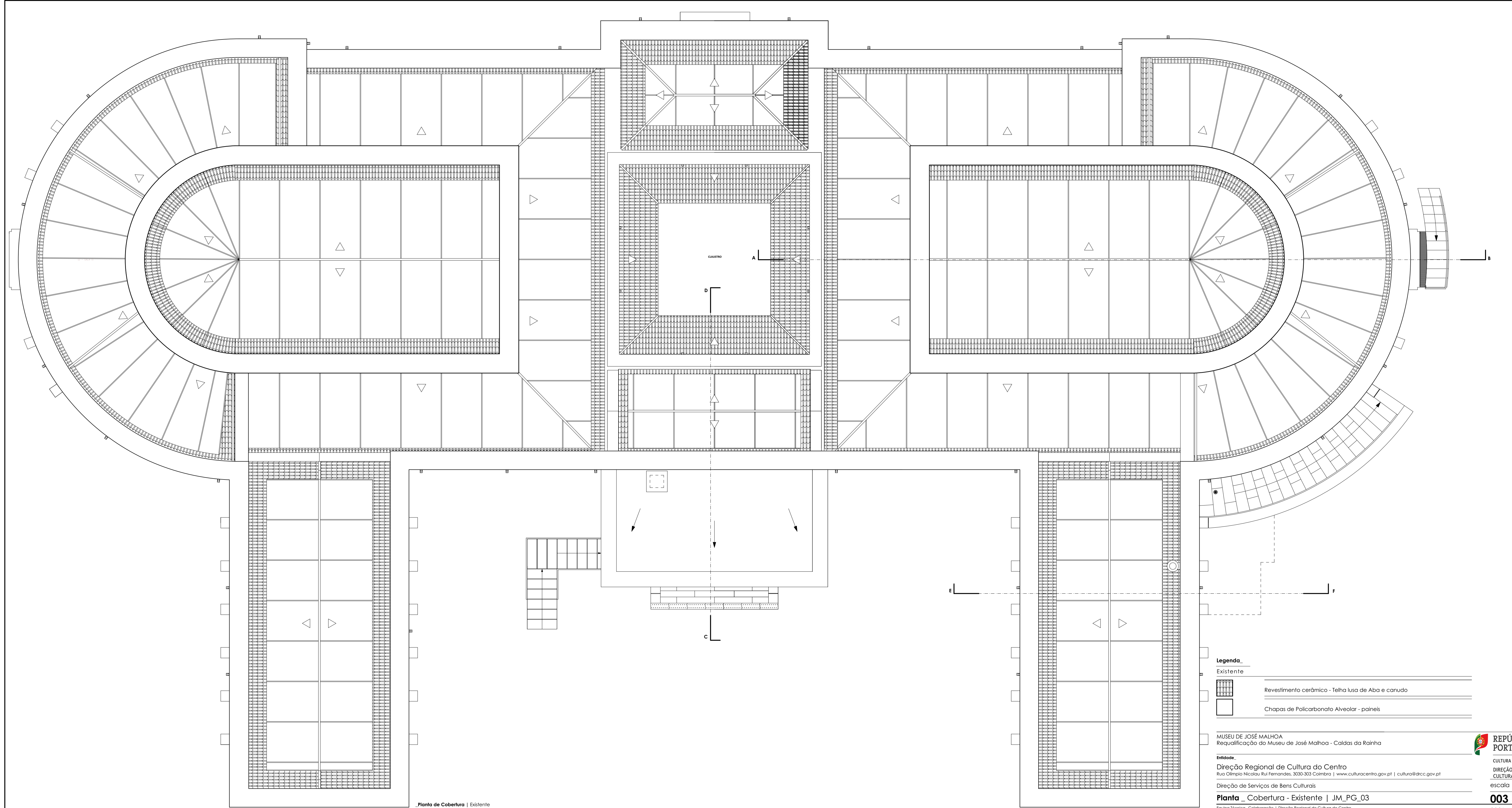
Planta de Cobertura | Existente
