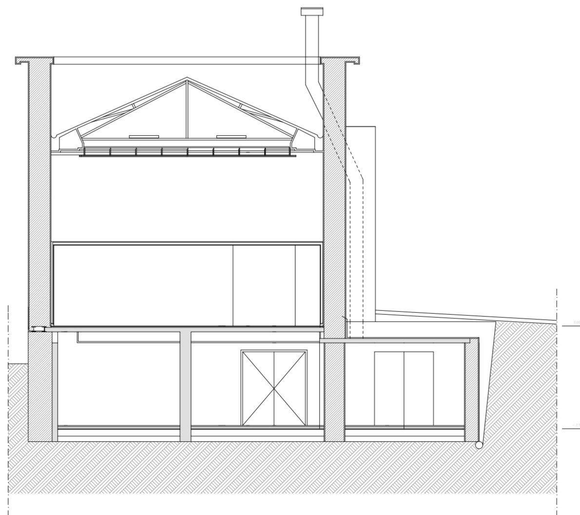
_Corte EF | Existente
