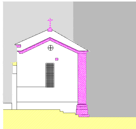
Alçado SUL
