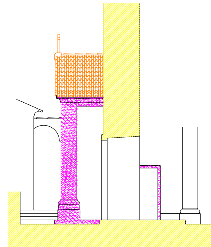
Alçado NASCENTE
