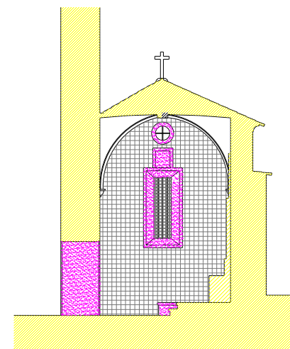
CORTE 1.1
