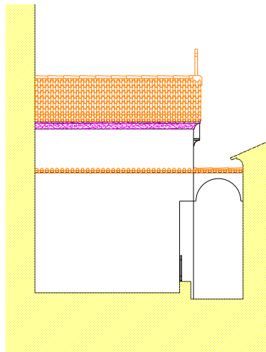
Alçado POENTE
