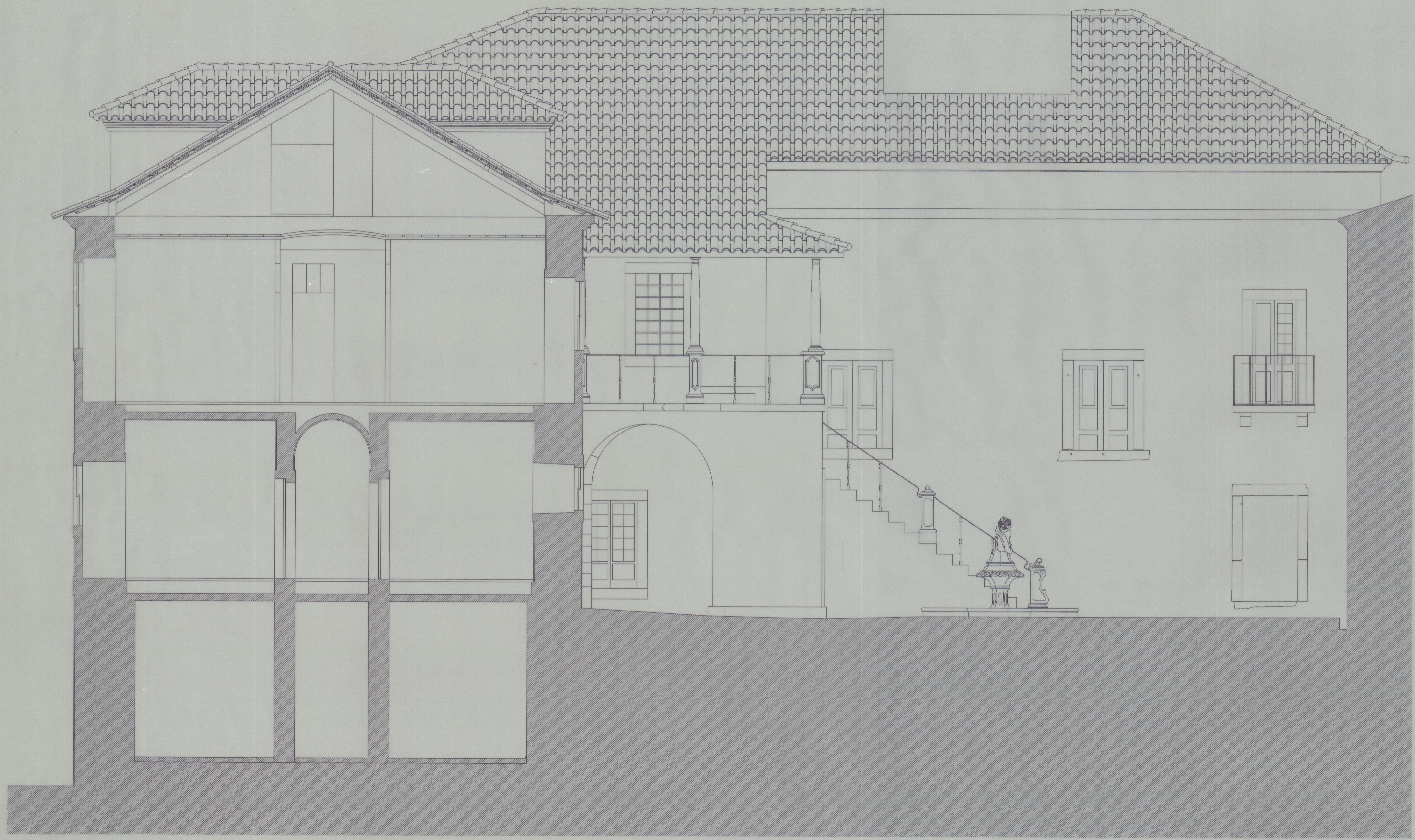
CORTE 1
