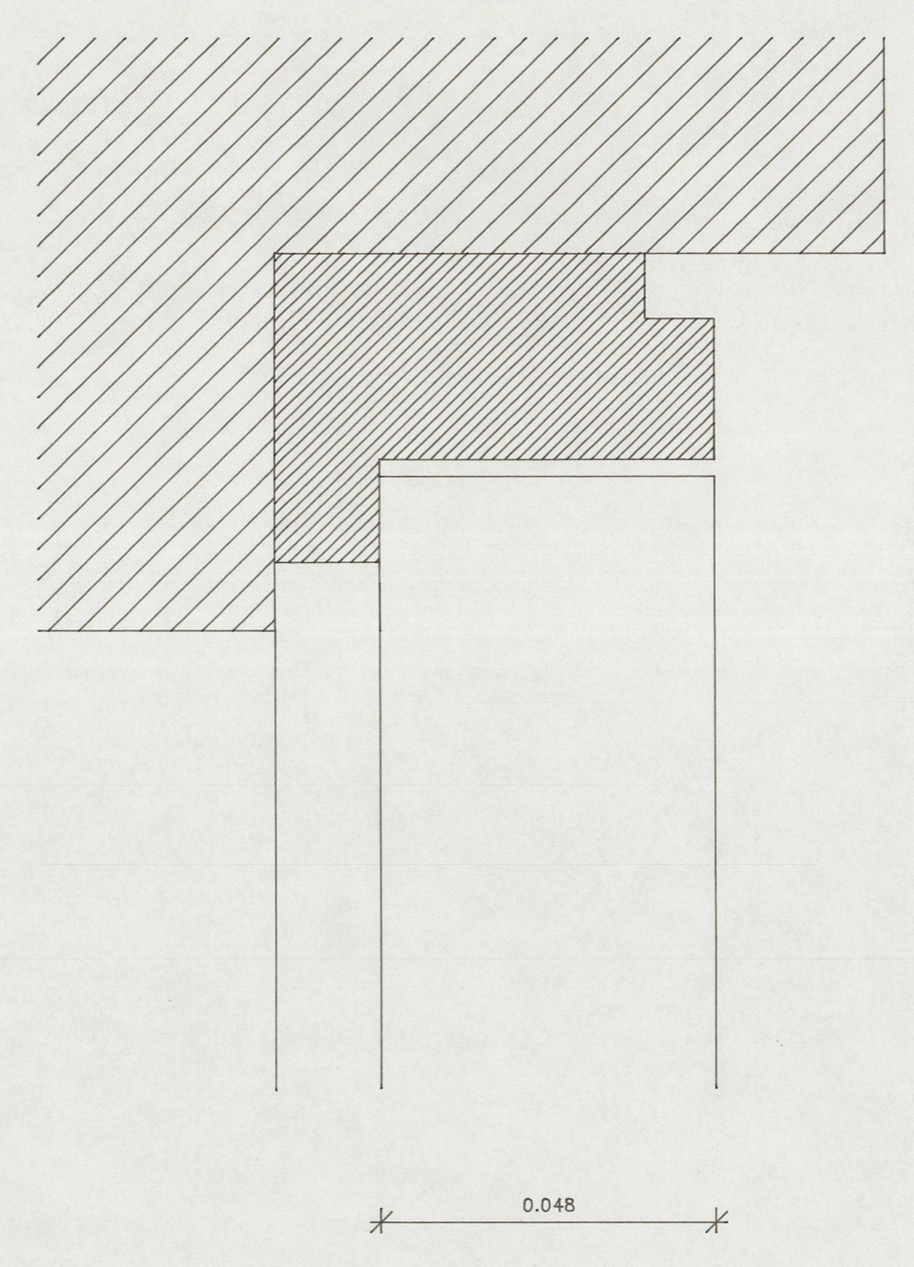
PORM. 2 esc. 1:1
