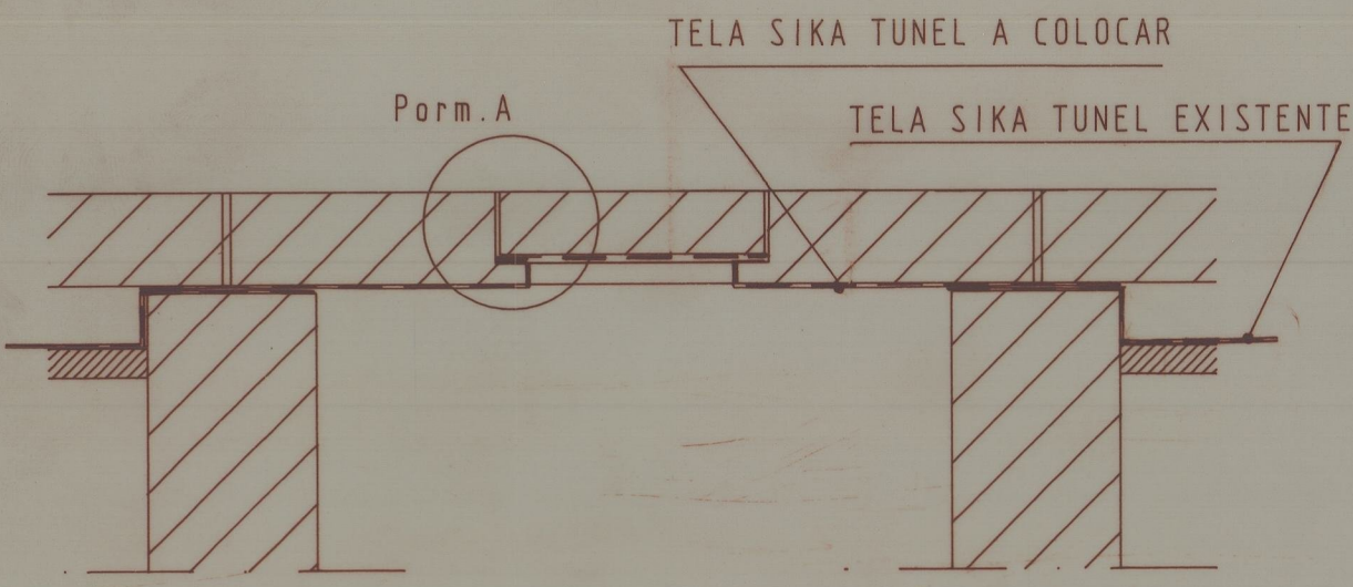
POÇO EXISTENTE (Impermeabilização da tampa)
