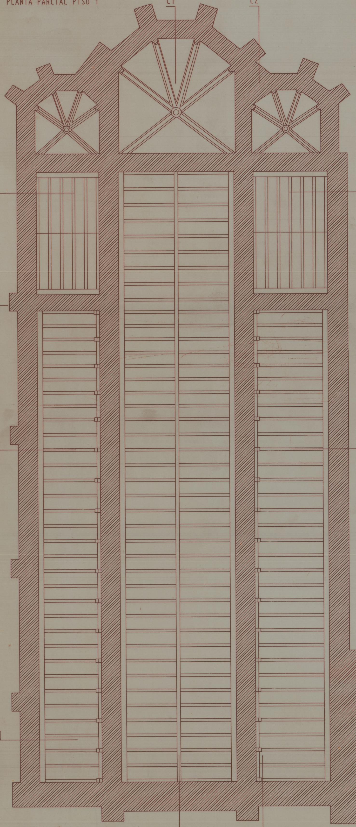
PLANTA DE TECTOS
