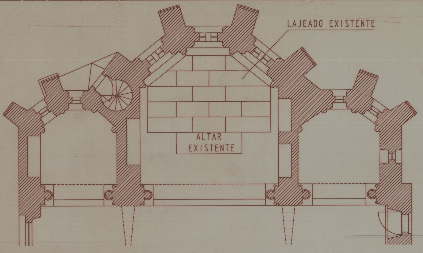
PLANTA PARCIAL PISO 1
