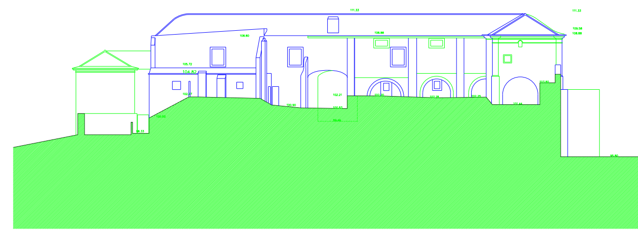
CORTE G.H
