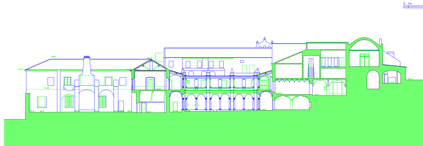
CORTE N.0
