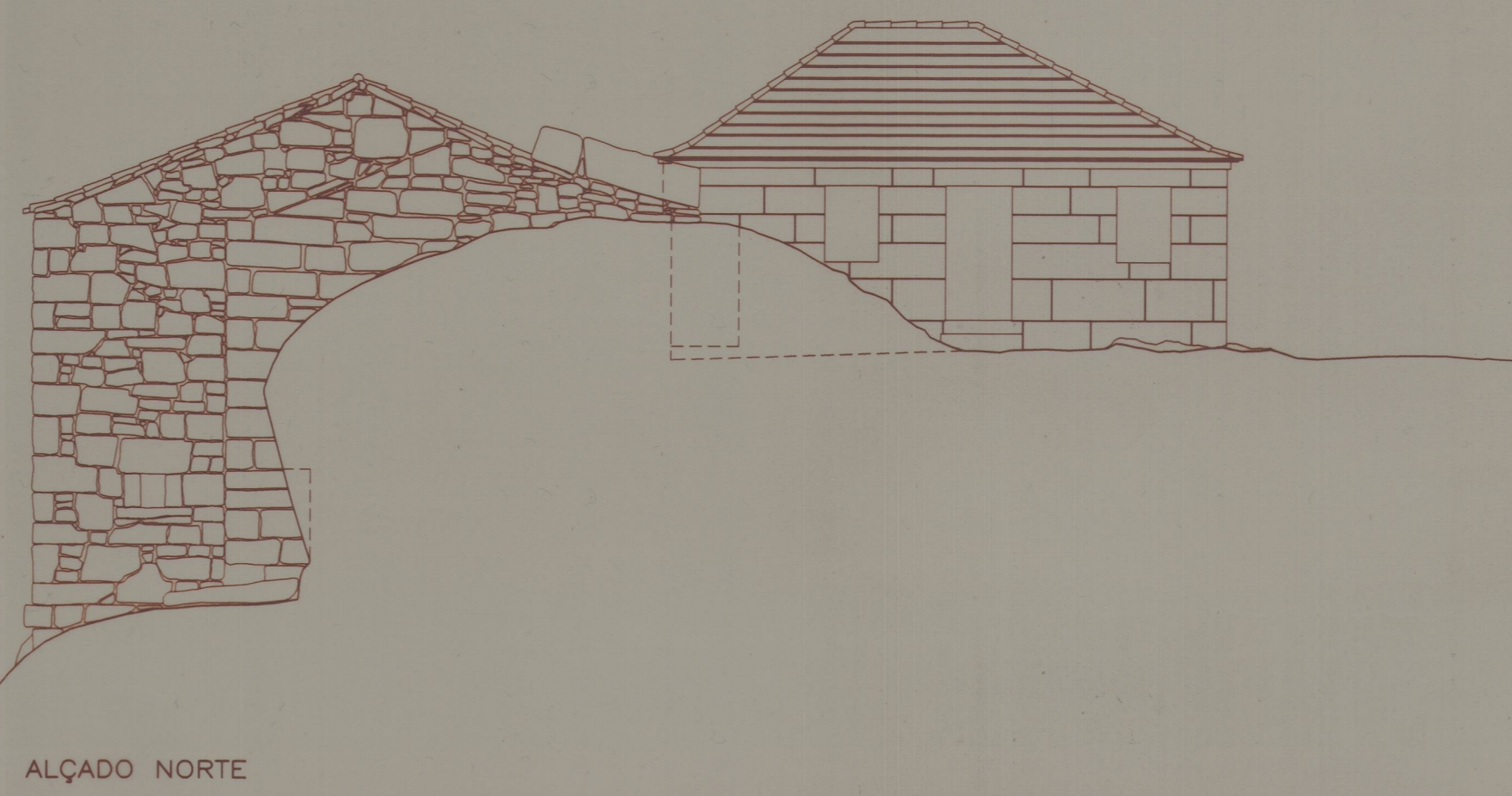
ALÇADO NORTE
