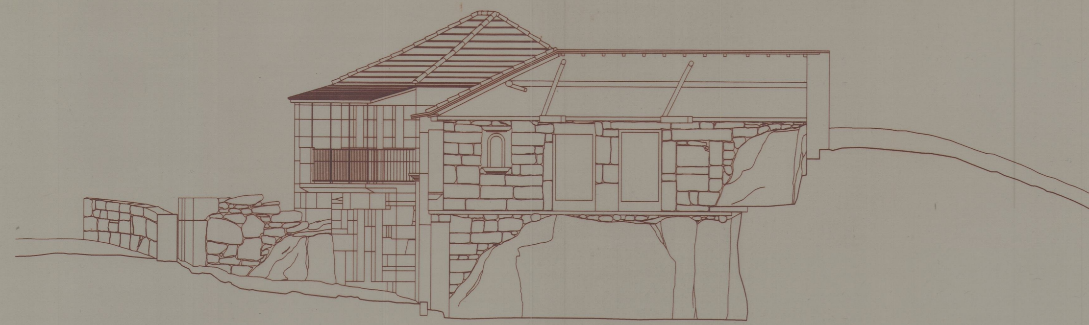
CORTE AB
