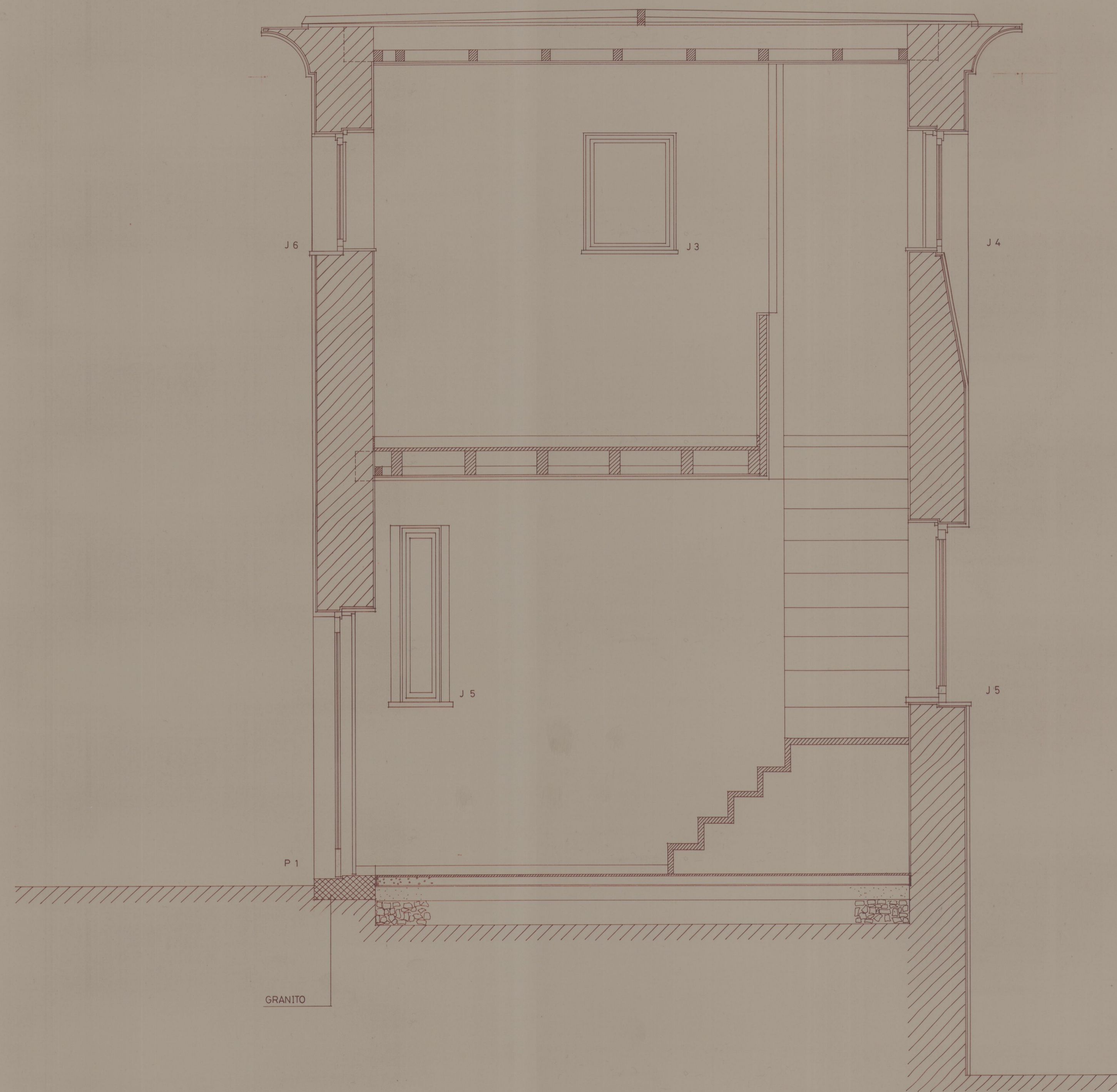
CORTE BB ESC. 1/20
