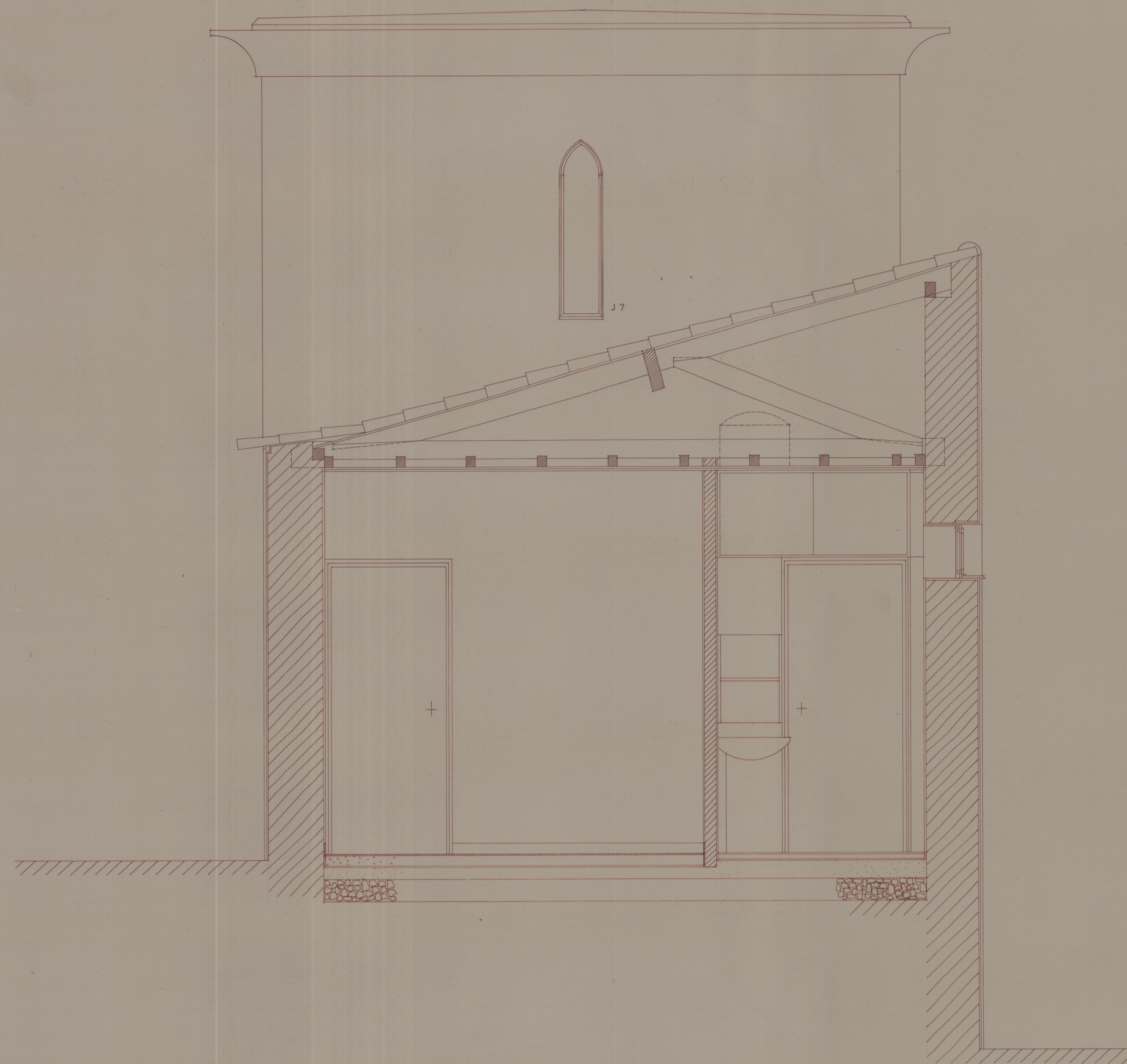
CORTE AA ESC. 1/20
