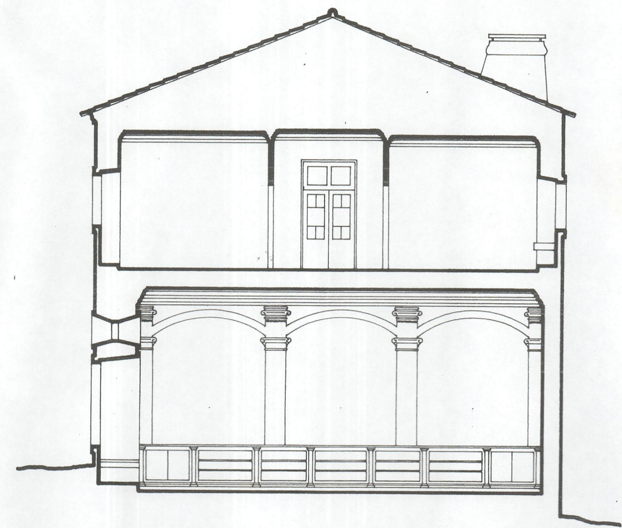
CORTE TRANSVERSAL A - B
