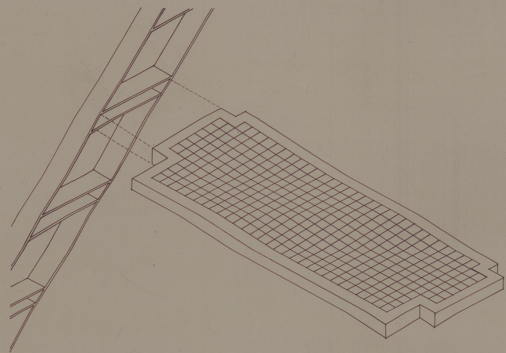
AXONOMETRIA DE DEGRAU TIPO
