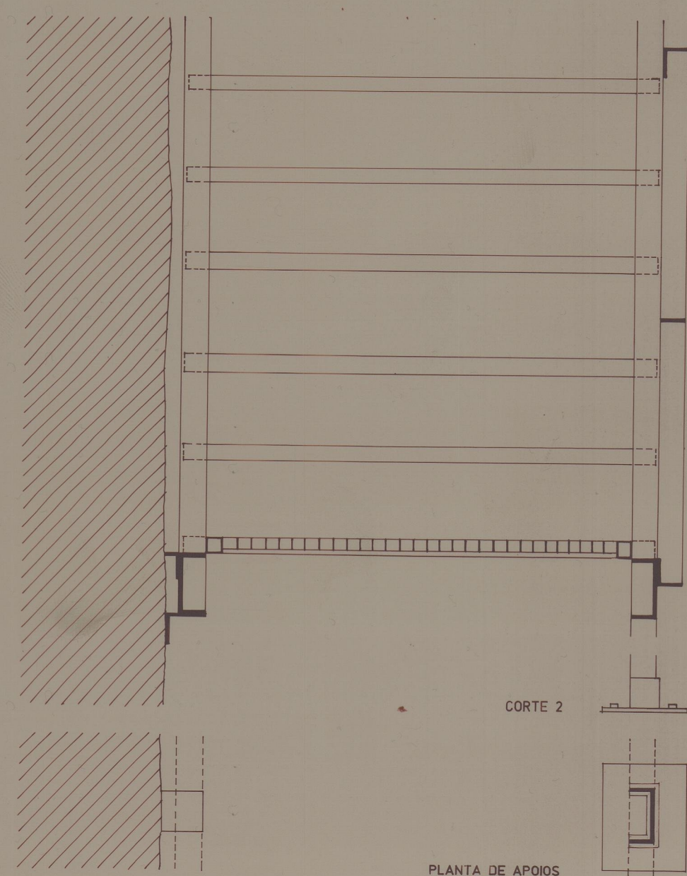
PLANTA DE APOIOS
