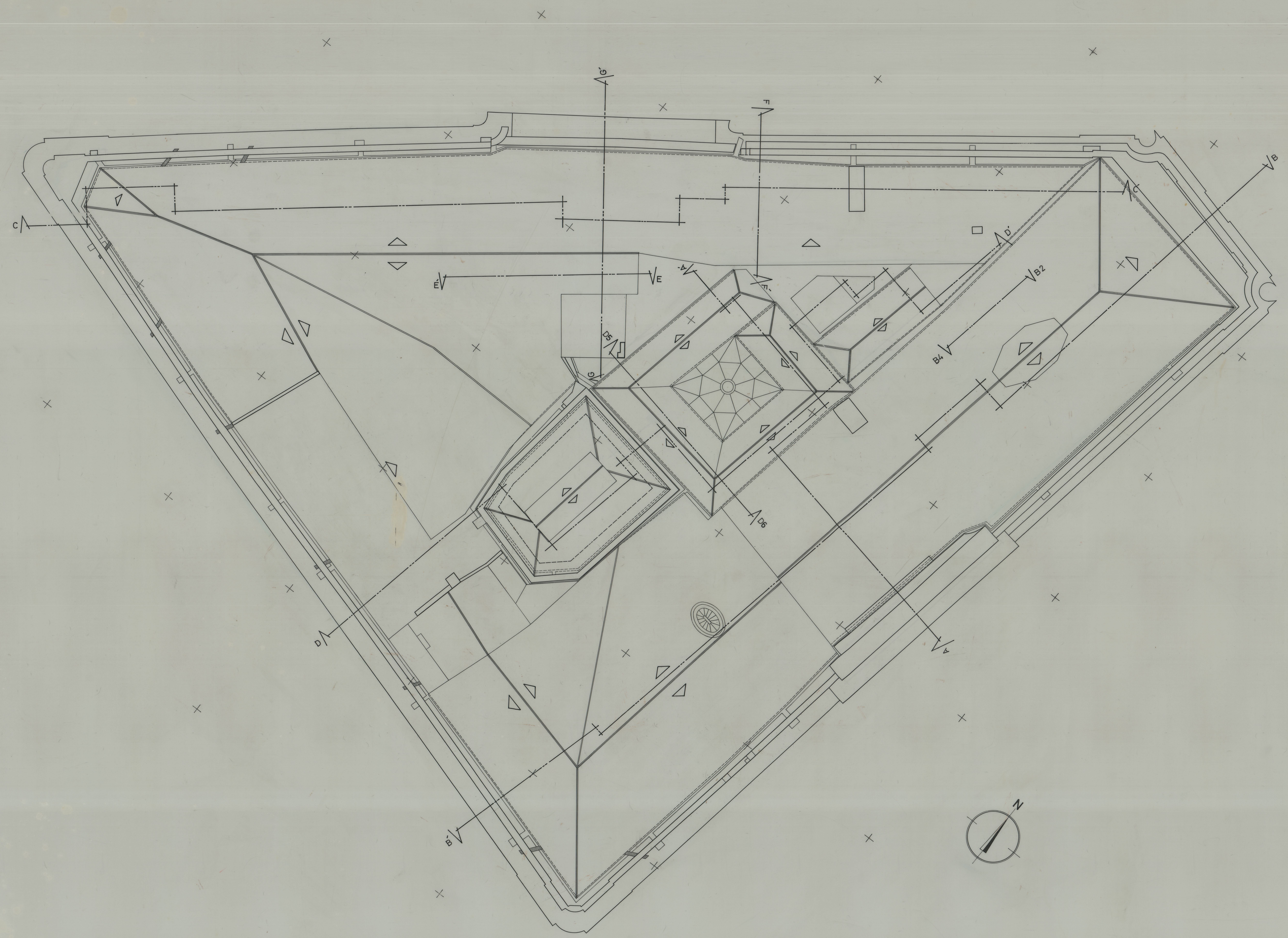
PLANTA DA COBERTURA
