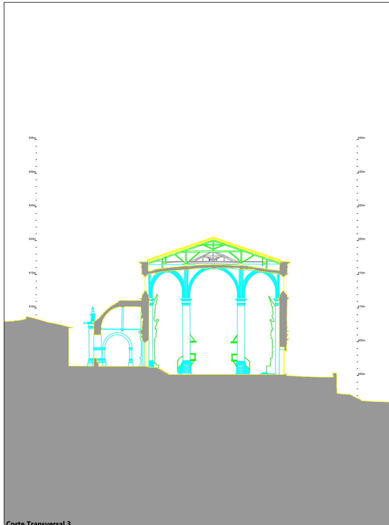
Corte Transversal 3
