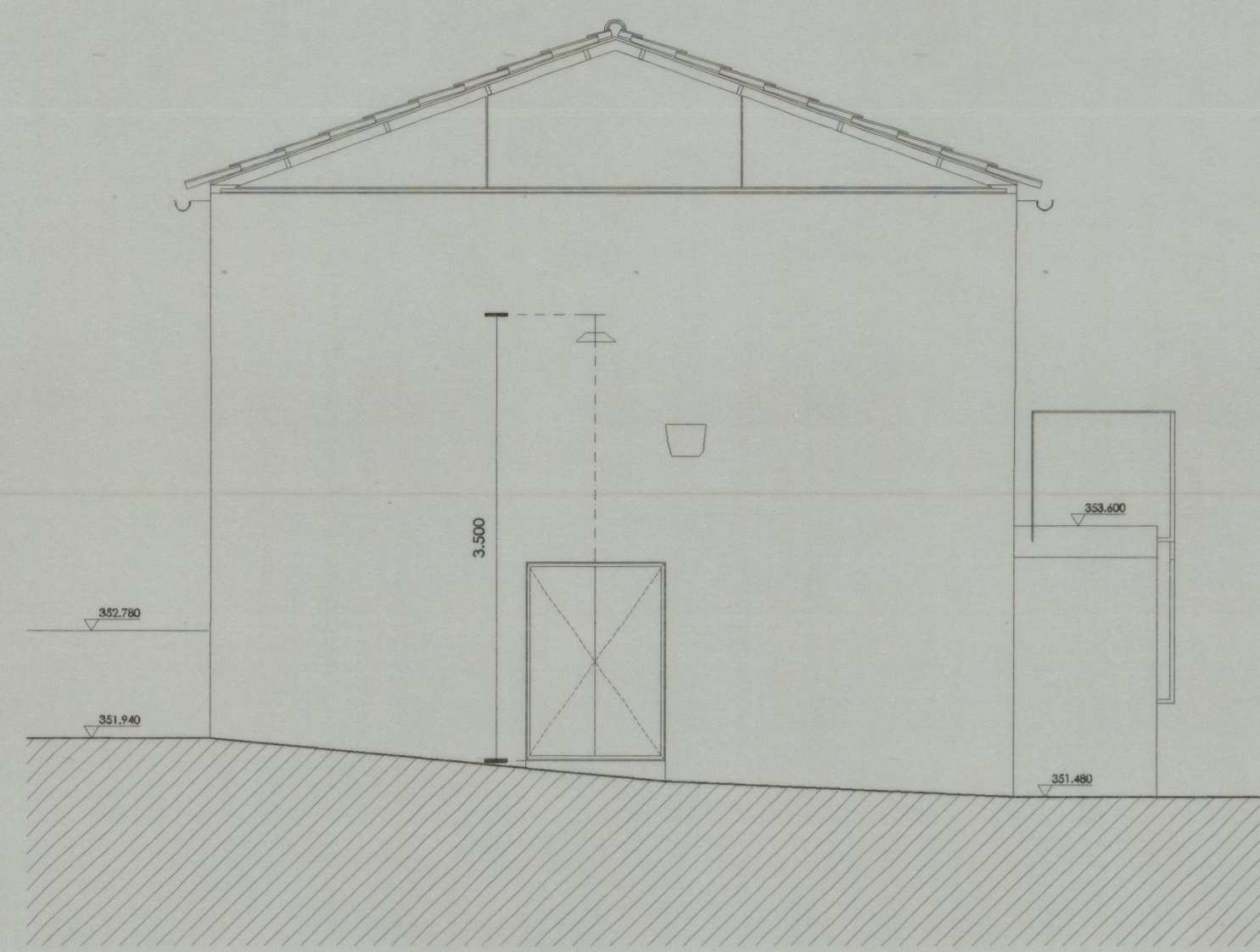
Alçado nordeste
