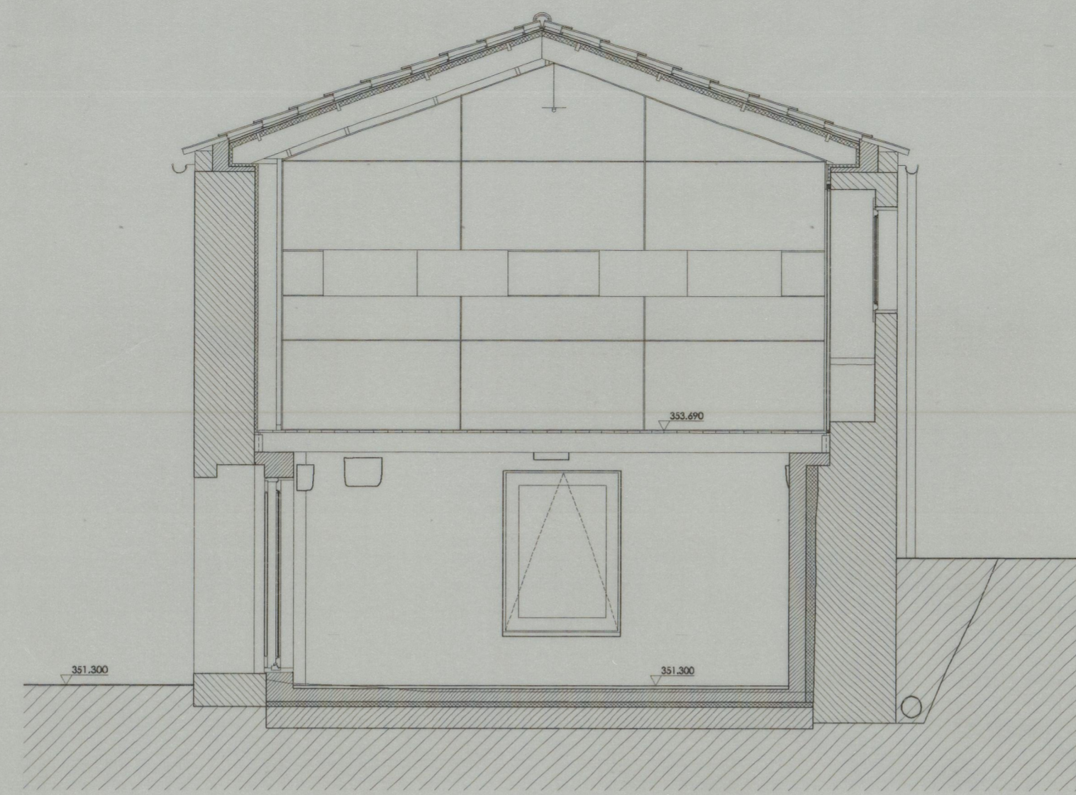
Corte C-C
