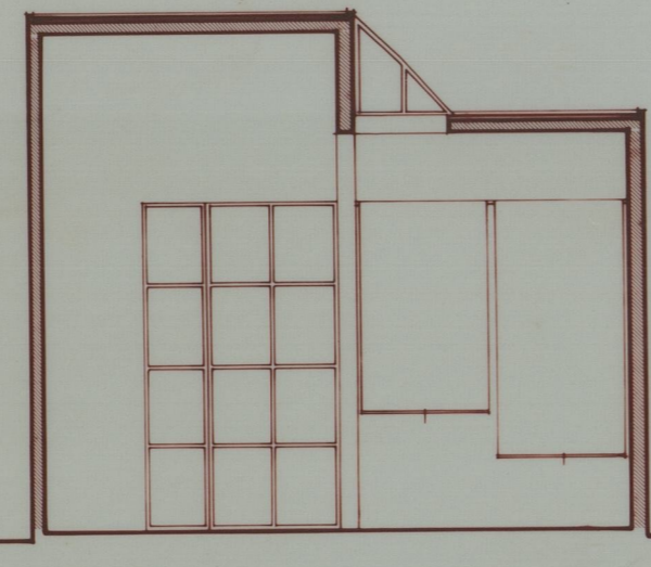
CORTE C-D
