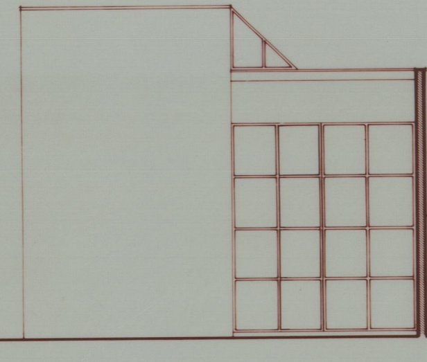
ALÇADO LAT DIREITO
