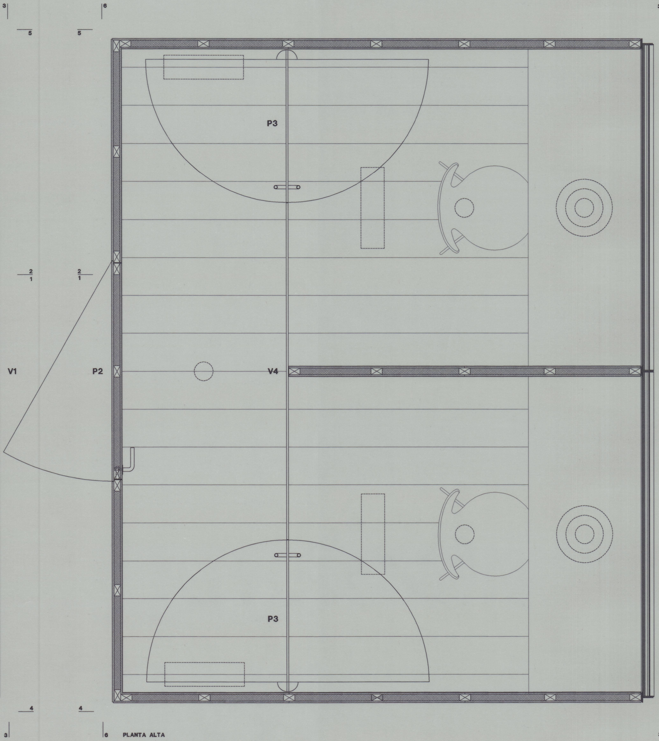
6 PLANTA ALTA
