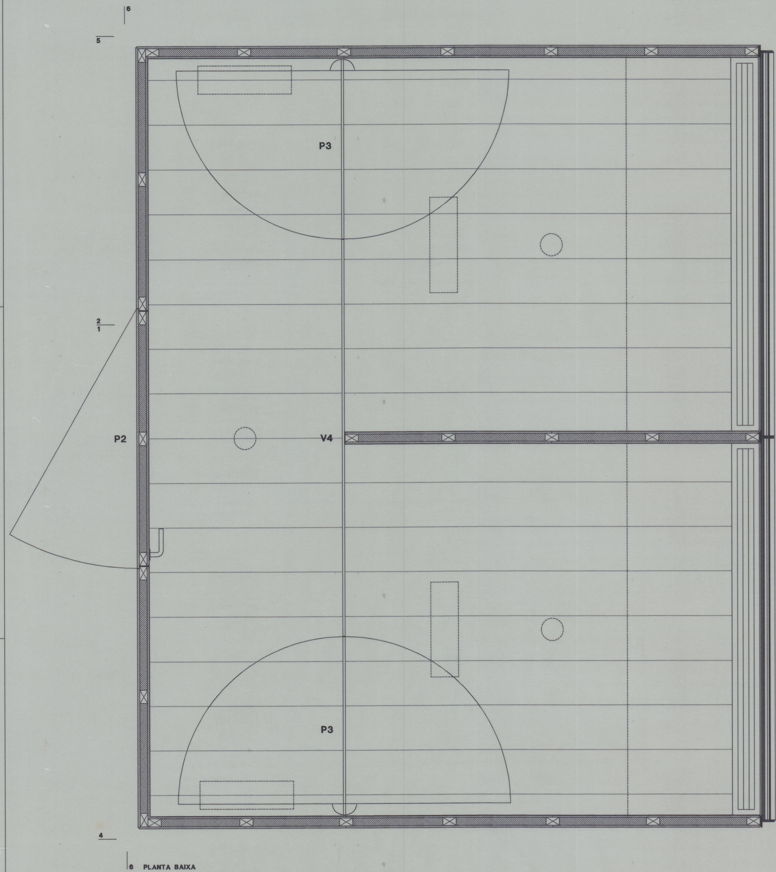
6 PLANTA BAIXA
