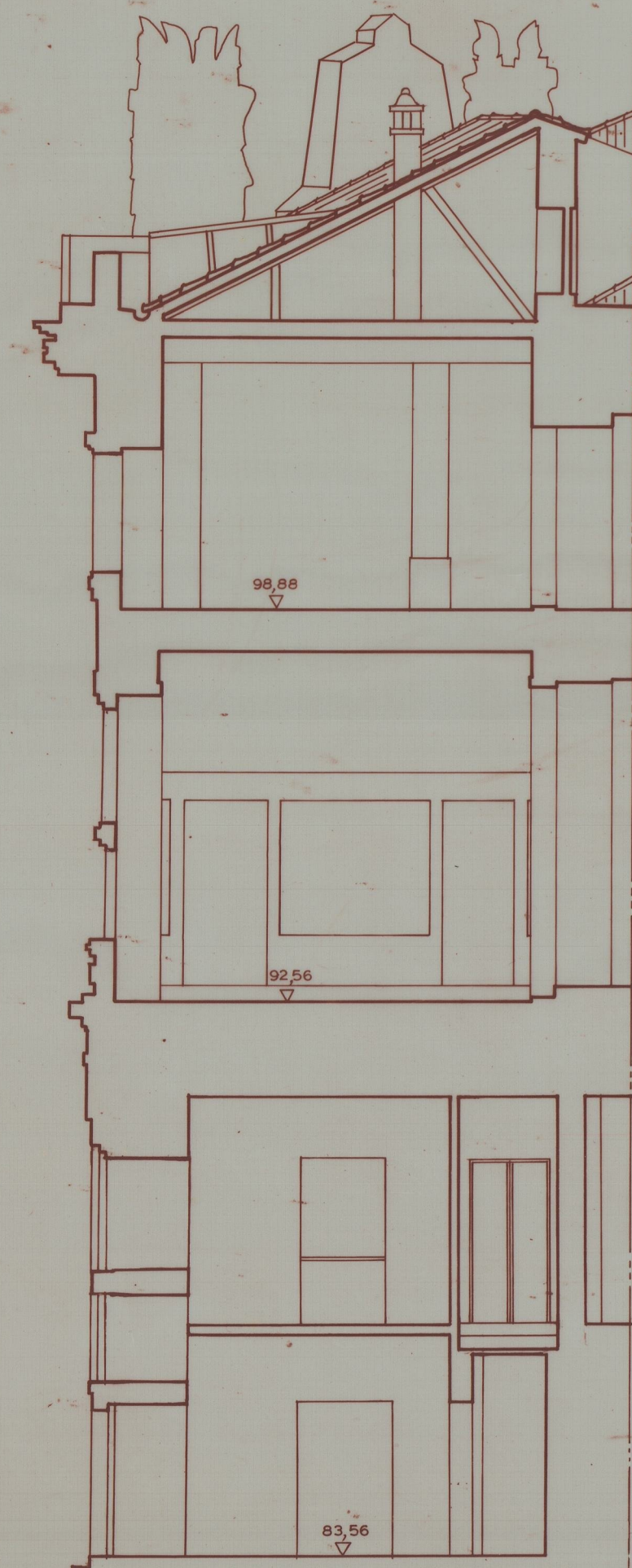
CORTE F-F'
