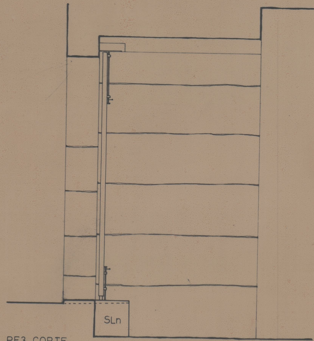
PF3 CORTE
