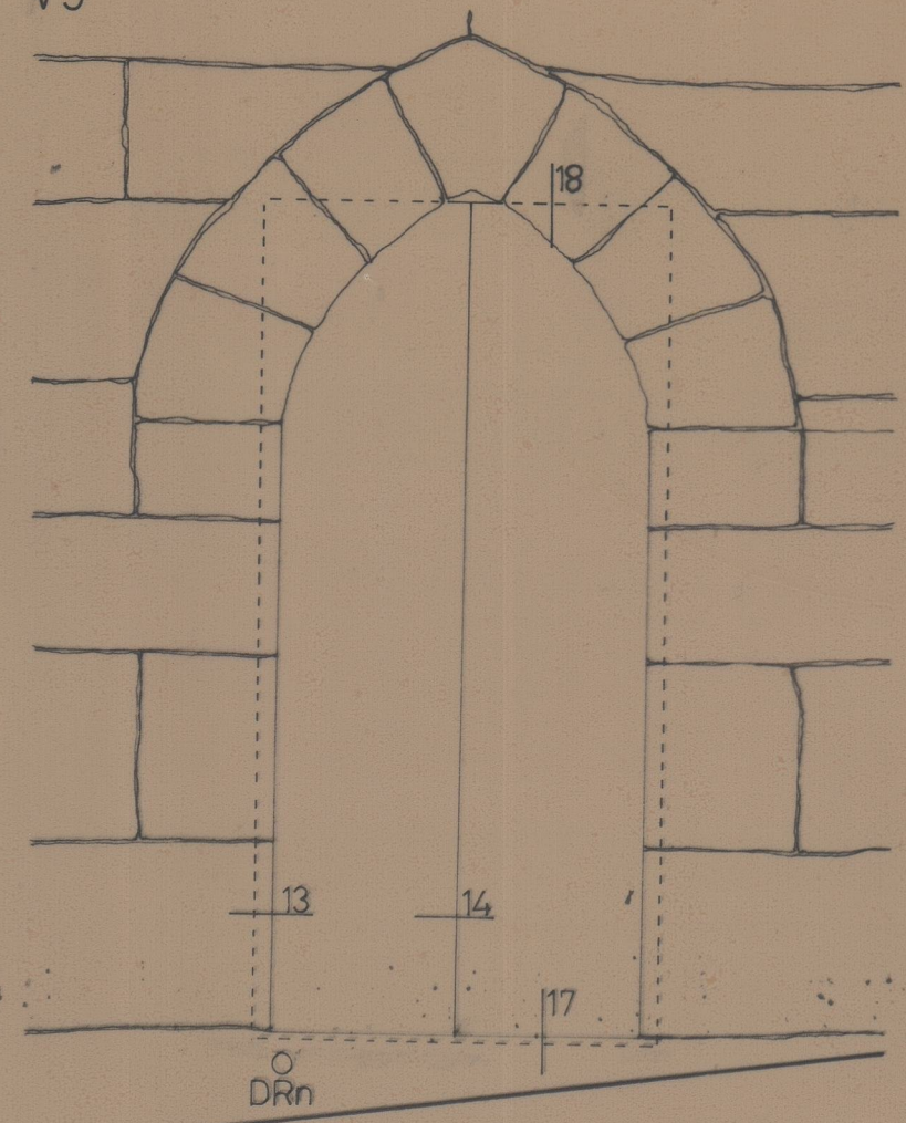
PF2 ALÇADO EXT.
