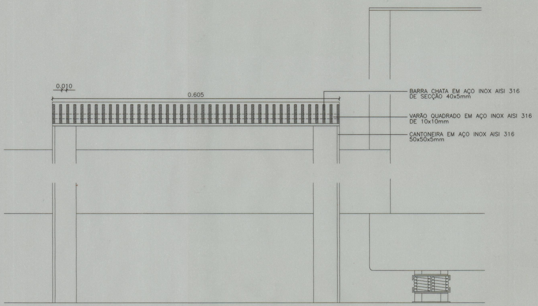
CORTE 1
