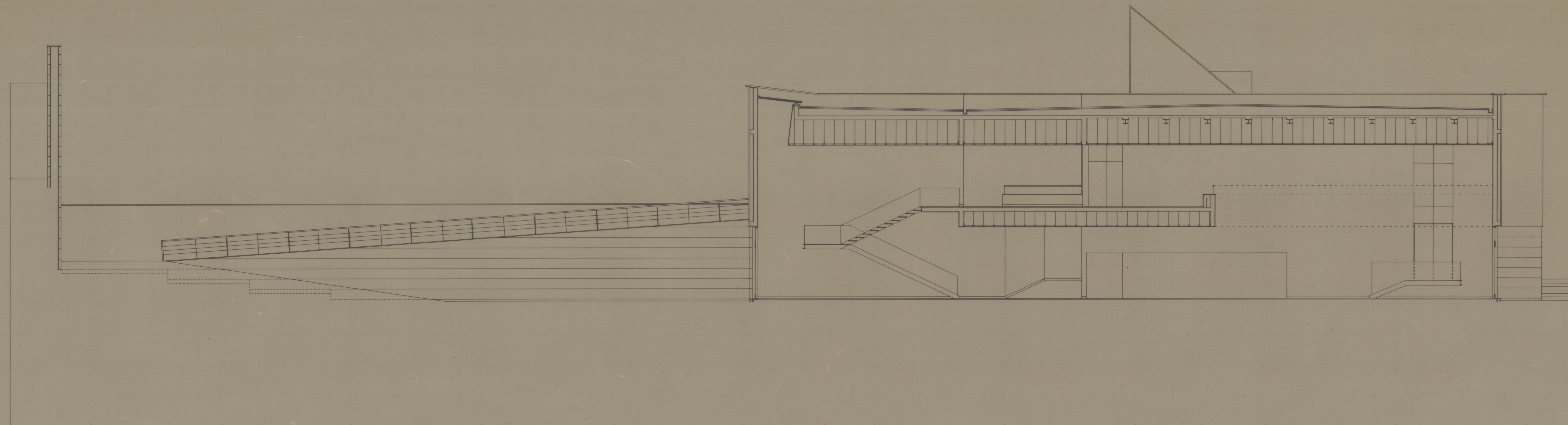
CORTE/ALÇADO 11'
